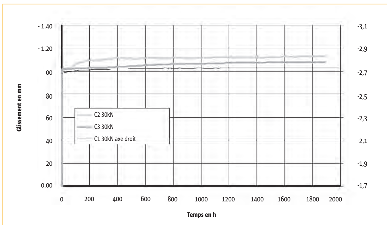
Fluage-adhérence après préchargement à f_b = 7.5 MPa; 60°C, béton à saturation constante
