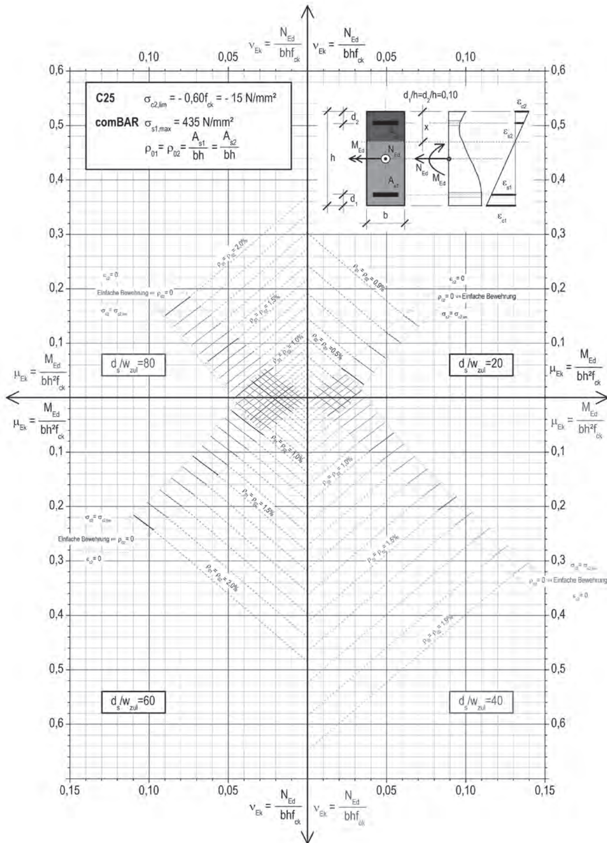
Graphique 2 : Renforcement anti-fissuration pour M_{Ed} + N_{Ed} ; C 25/30; d/h = 0,10
