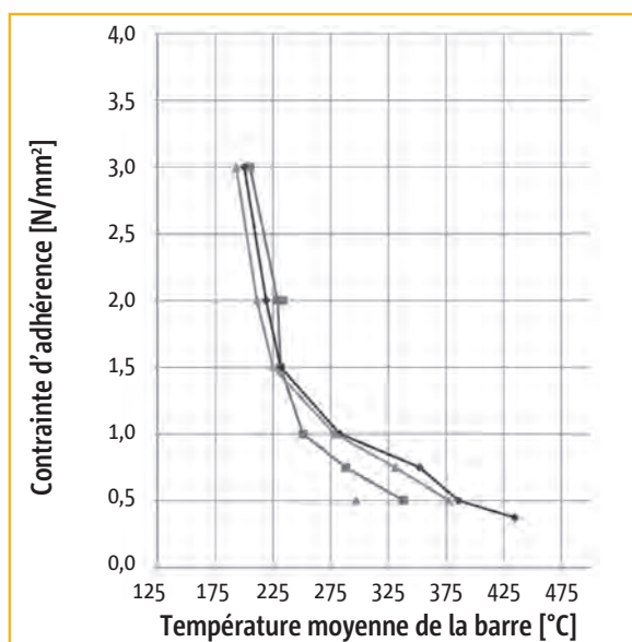
La contrainte d'adhérence en fonction de la température moyenne
