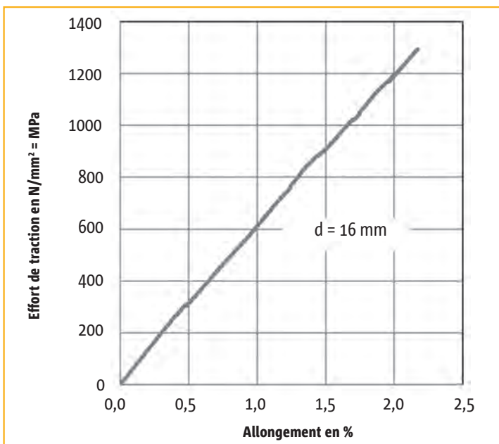
Diagramme contrainte-déformation
