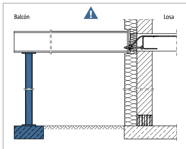
Fig. 162: Schöck Isokorb® T tipo SQ: Se requiere apuntalamiento continuo
