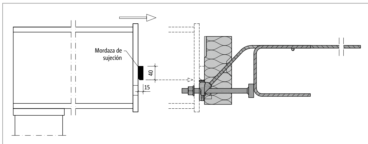
Fig. 160: Schöck Isokorb® T tipo SQ: Montaje de la viga de acero
