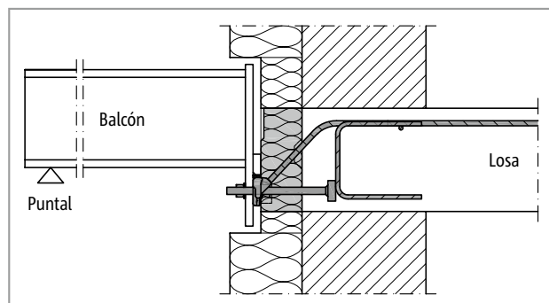
Fig. 137: Schöck Isokorb® T tipo SQ: Paso sin barreras por desplazamiento de altura
