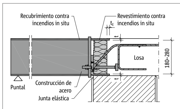
Fig. 154: Schöck Isokorb® T tipo SQ: Revestimiento contra incendios in situ T tipo SQ, construcción de acero con recubrimiento contra incendios; sección
