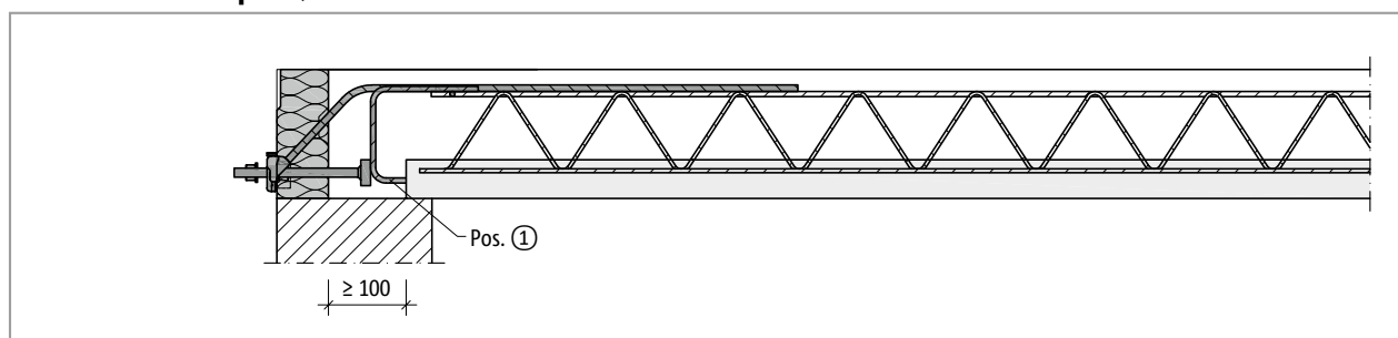
Fig. 157: Schöck Isokorb® T tipo SQ: Armadura in situ para sistema de construcción con prefabricados, sección
