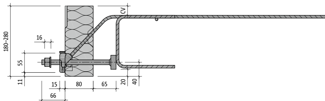
Fig. 151: Schöck Isokorb® T tipo SQ-V1: Sección del producto
