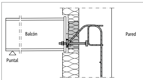
Fig. 138: Schöck Isokorb® T tipo SQ-WU: Construcción especial; necesaria en caso de conexión a un muro de hormigón armado con un espesor mínimo de 200 mm
