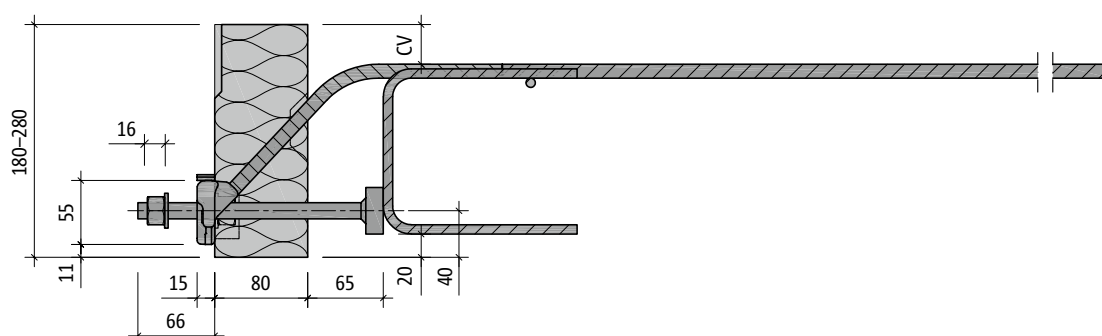
Fig. 153: Schöck Isokorb® T tipo SQ-V3: Sección del producto
