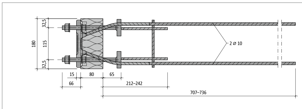
Fig. 149: Schöck Isokorb® T tipo SQ-V2: Plano
