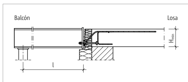
Fig. 142: Schöck Isokorb® T tipo SQ: Sistema estático
