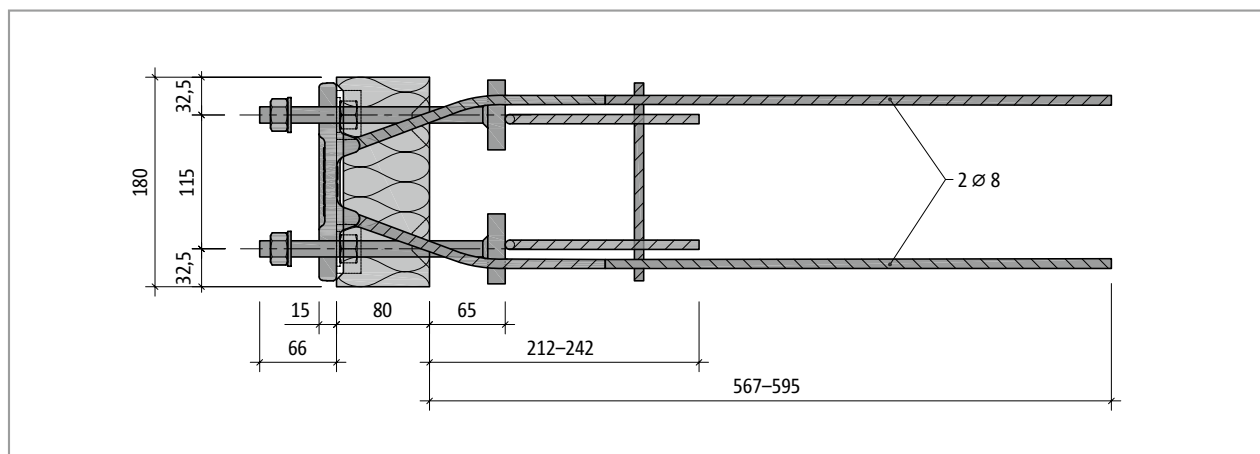
Fig. 148: Schöck Isokorb® T tipo SQ-V1: Plano
