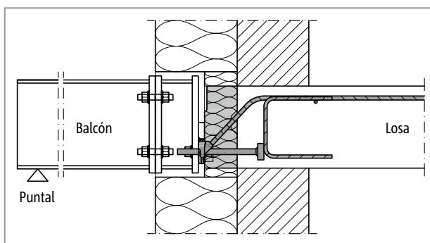
Fig. 140: Schöck Isokorb® T tipo SQ: Conexión del soporte de acero a un adaptador que compensa el espesor del aislamiento exterior
