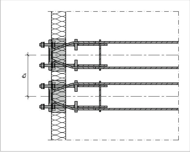
Fig. 147: Schöck Isokorb® T tipo SQ: Distancia entre ejes
