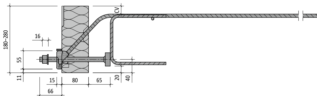
Fig. 152: Schöck Isokorb® T tipo SQ-V2: Sección del producto
