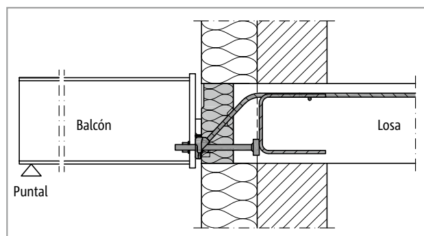
Fig. 139: Schöck Isokorb® T tipo SQ: Con ayuda del saliente de la losa, el elemento aislante cierra al ras con el aislamiento del muro. Aquí se deberán tener en cuenta las distancias laterales al borde
