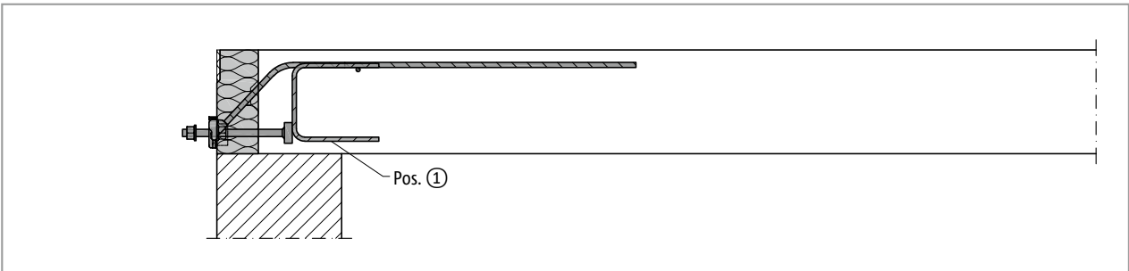
Fig. 155: Schöck Isokorb® T tipo SQ: Armadura in situ, sección
