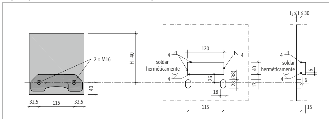
Fig. 159: Schöck Isokorb® T tipo SQ: Construcción de la conexión de la placa frontal
