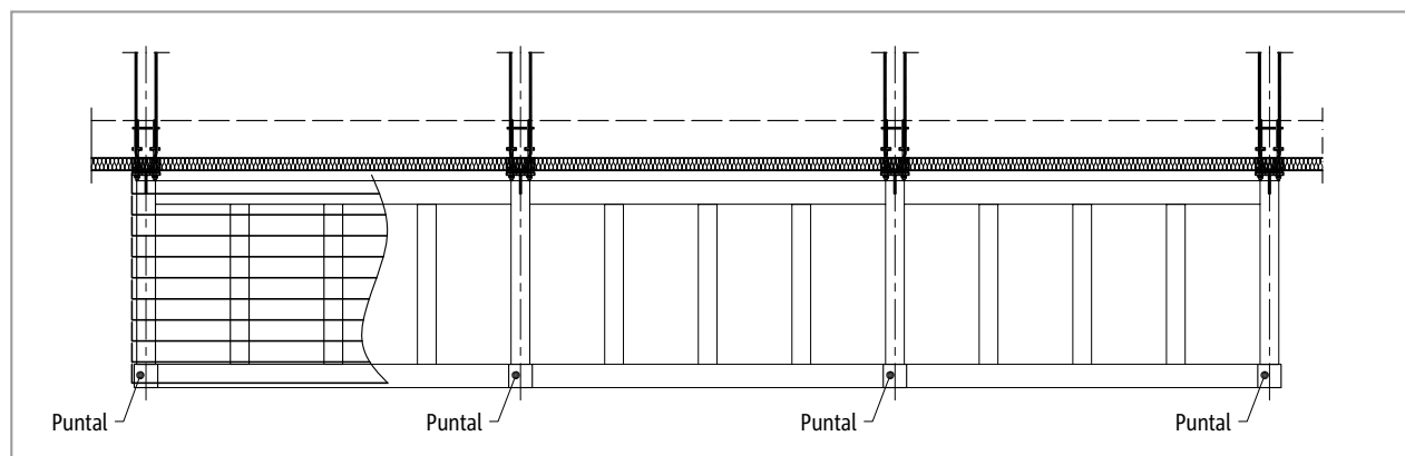
Fig. 134: Schöck Isokorb® T tipo SQ: Balcón apoyado en puntales
