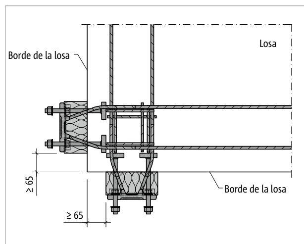
Fig. 146: Schöck Isokorb® T tipo SQ: Distancias al borde en el esquinero externo en caso de Isokorb® dispuestos perpendicularmente entre sí
