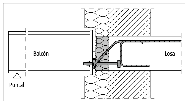
Fig. 135: Schöck Isokorb® T tipo SQ: Conexión a la losa de hormigón armado; elemento aislante dentro del aislamiento externo
