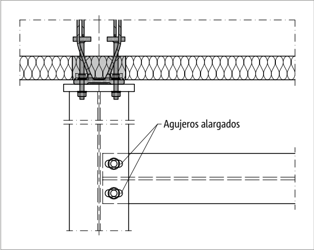
Fig. 144: Schöck Isokorb® T tipo SQ: Detalle de la fuga de expansión que permite el desplazamiento en caso de dilatación por temperatura
