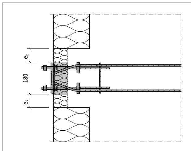
Fig. 145: Schöck Isokorb® T tipo SQ: Distancias al borde
