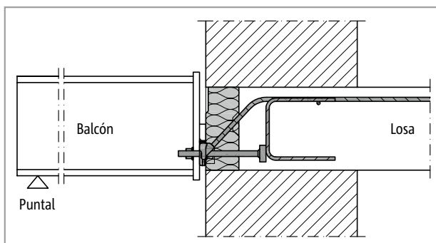
Fig. 136: Schöck Isokorb® T tipo SQ: Conexión a la losa de hormigón armado; construcción monolítica del muro
