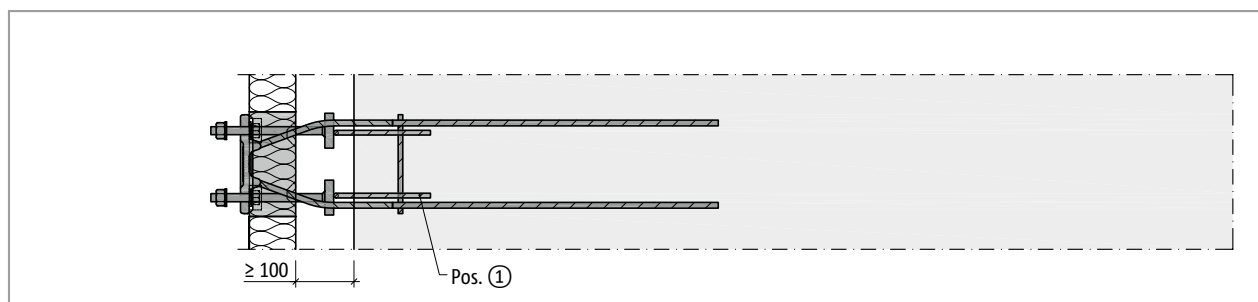
Fig. 158: Schöck Isokorb® T tipo SQ: Armadura in situ para sistema de construcción con prefabricados, plano
