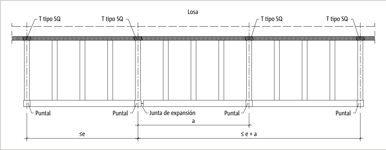
Fig. 143: Schöck Isokorb® T tipo SQ: Separación máxima de las juntas de expansión e y saliente lateral a
