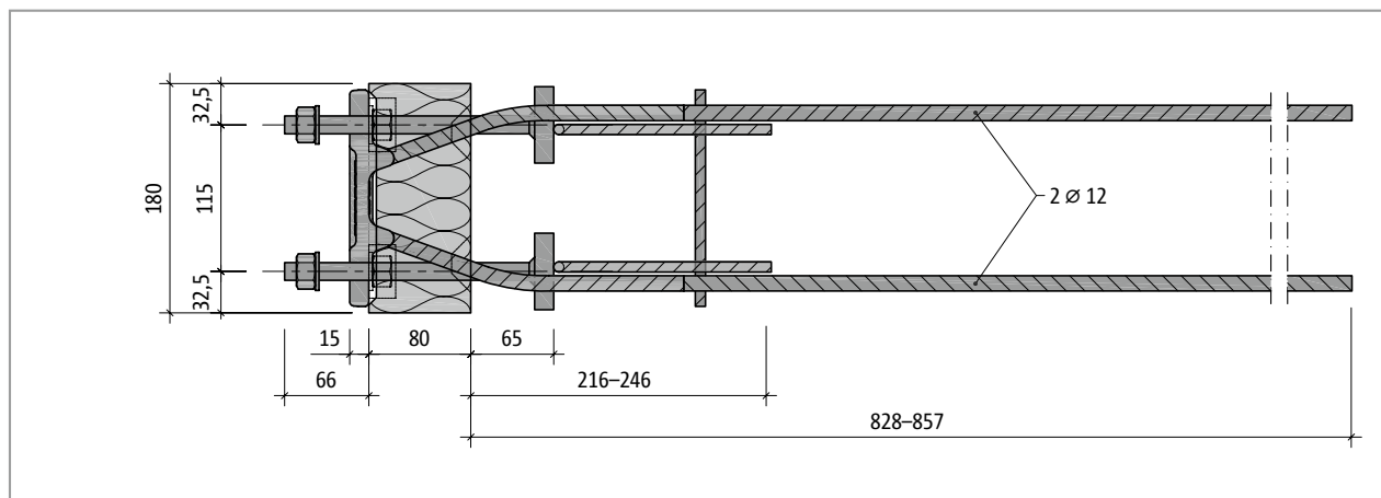
Fig. 150: Schöck Isokorb® T tipo SQ-V3: Plano
