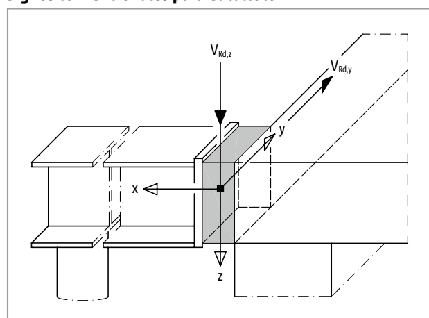
Fig. 141: Schöck Isokorb® T tipo SQ: Signos convencionales para el cálculo
