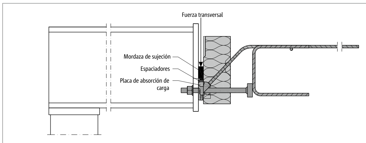
Fig. 161: Schöck Isokorb® T tipo SQ: Mordaza de sujeción in situ para la transferencia de la fuerza transversal
