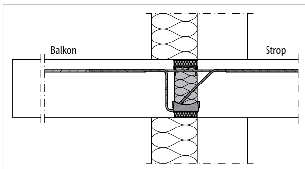
Ilustr. 40: Schöck Isokorb® T typu KL: Balkon przy ścianie z izolacją zewnętrzną
