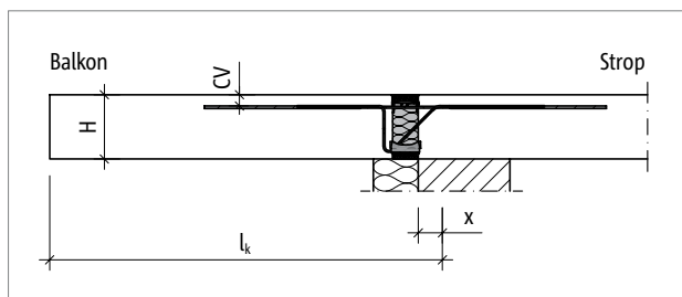
Ilustr. 44: Schöck Isokorb® T typu K: Schemat statyczny
