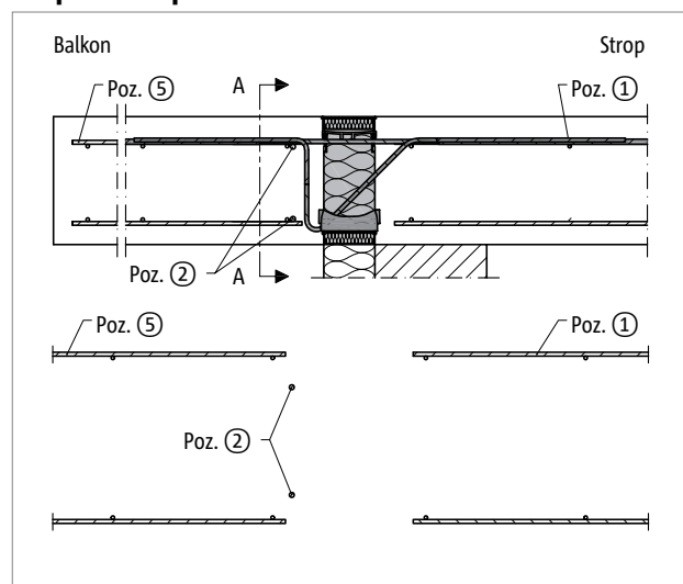
Ilustr. 51: Schöck Isokorb® T typu KL: Zbrojenie na budowie przy podparciu bezpośrednim
