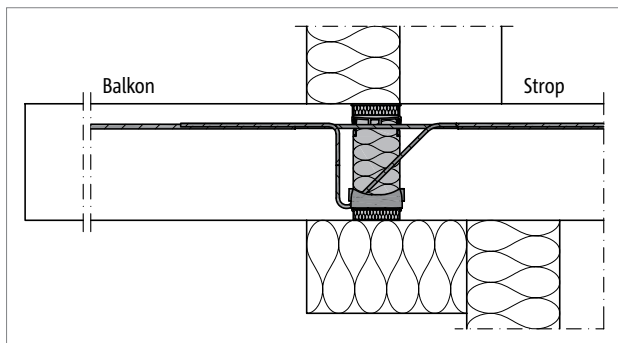
Ilustr. 42: Schöck Isokorb® T typu KL: Balkon przy przesuniętej krawędzi stropu i ścianie z izolacją zewnętrzną
