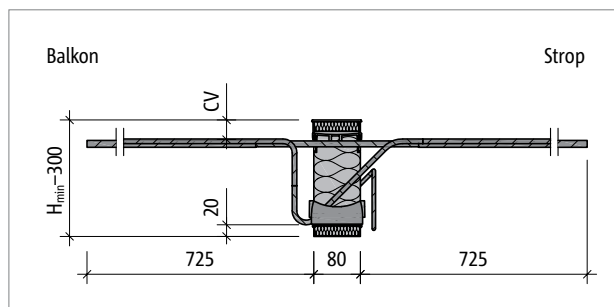
Ilustr. 46: Schöck Isokorb® T typu KL-M8 do M12: Przekrój
