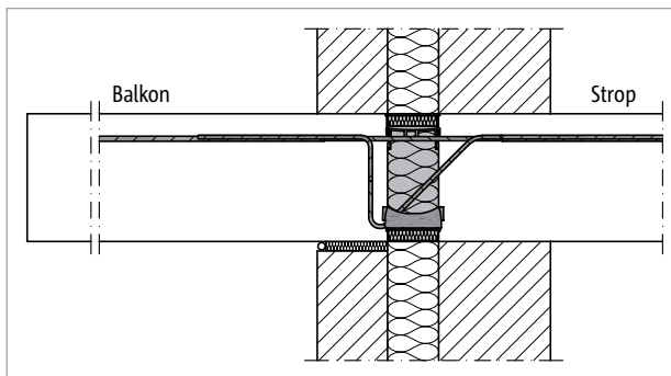
Ilustr. 43: Schöck Isokorb® T typu KL: Połączenie przy ścianie murowanej dwuwarstwowej z izolacją
