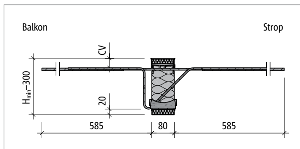
Ilustr. 45: Schöck Isokorb® T typu KL-M1 do M7-V1/V2: Przekrój
