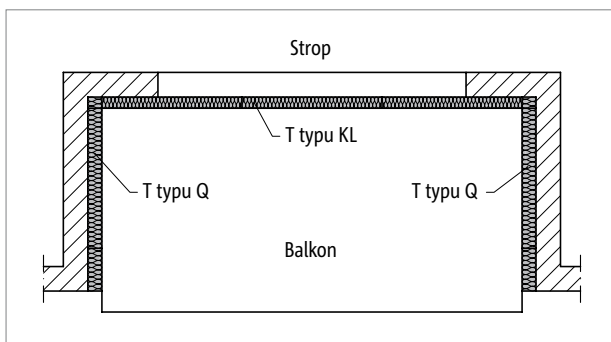
Ilustr. 37: Schöck Isokorb® T typu KL i typu Q: Balkon podparty trójkątnie
