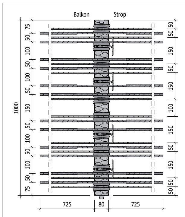
Ilustr. 48: Schöck Isokorb® T typu KL-M10-V2: Rzut poziomy
