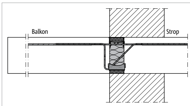
Ilustr. 41: Schöck Isokorb® T typu KL: Balkon przy ścianie jednowarstwowej
