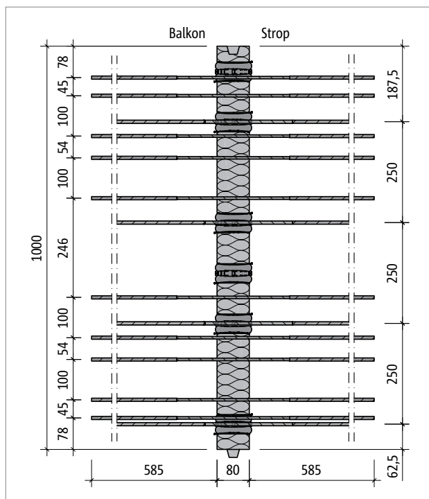
Ilustr. 47: Schöck Isokorb® T typu KL-M4-V1: Rzut poziomy
