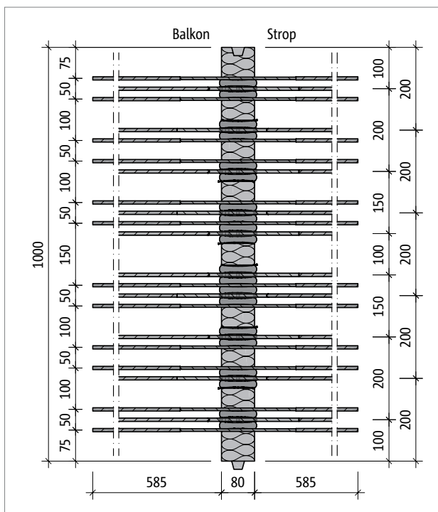
Ilustr. 50: Schöck Isokorb® T typu KL-M4-VV1: Rzut poziomy
