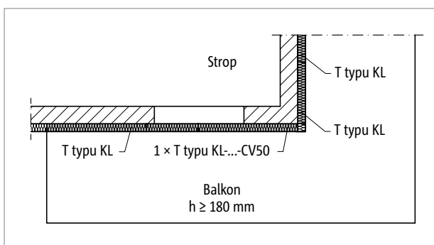
Ilustr. 39: Schöck Isokorb® T typu KL: Balkony narożne zewnętrzne
