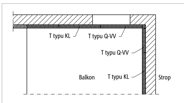
Ilustr. 38: Schöck Isokorb® T typu KL i Q-VV: Balkon podparty dwustronnie
