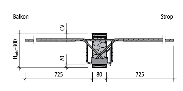
Ilustr. 49: Schöck Isokorb® T typu KL-M4-VV1: Przekrój
