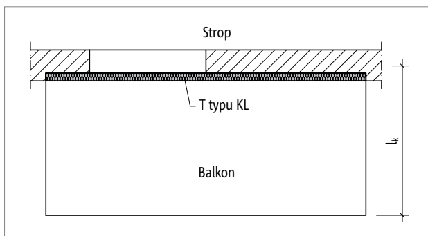
Ilustr. 36: Schöck Isokorb® T typu KL: Balkon wspornikowy
