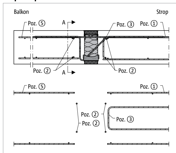
Ilustr. 52: Schöck Isokorb® T typu KL: Zbrojenie na budowie przy podparciu pośrednim
