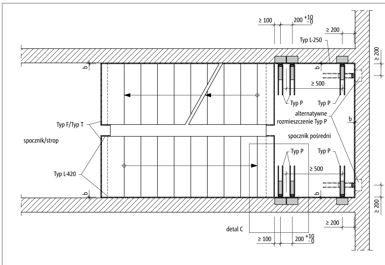
Ilustr. 107: Schöck Tronsole® typu P: Rozmieszczenie elementów z zastosowanym elementem Tronsole® typu L - rzut poziomy
