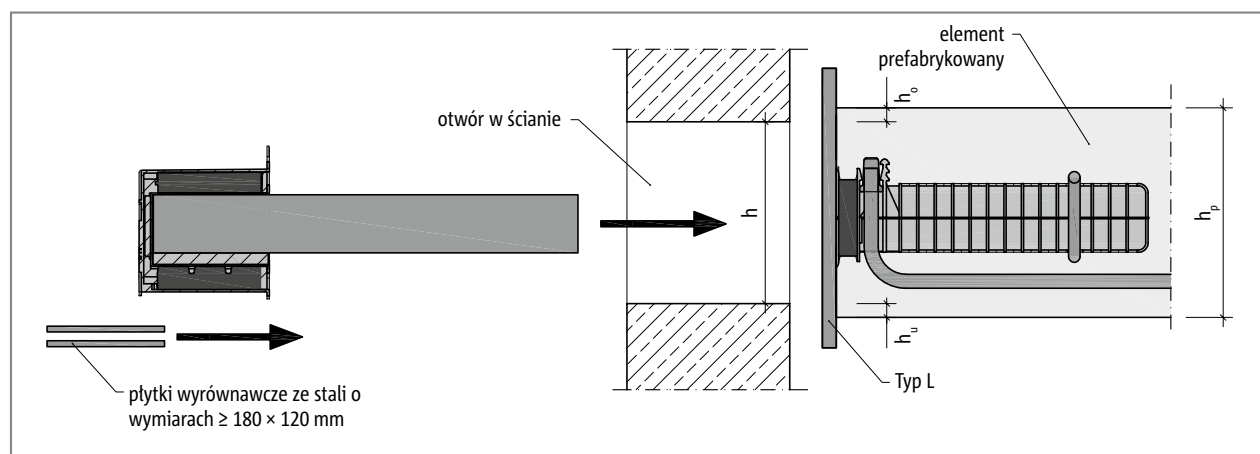
Ilustr. 122: Schöck Tronsole® typu P: Otwór w ścianie przy montażu elementów prefabrykowanych
