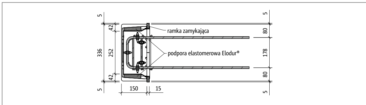
Ilustr. 139: Schöck Tronsole® typu Z-VH+VH-T: Przekrój poziomy
