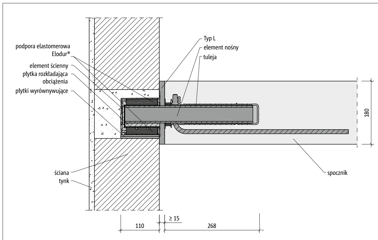
Ilustr. 101: Schöck Tronsole® typu P: Płyta spocznikowa prefabrykowana i Tronsole® typu L
