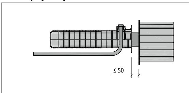
Ilustr. 70: Schöck Tronsole® typu Q: Wariant montażu dla szerokości szczeliny \leq 50 mm
