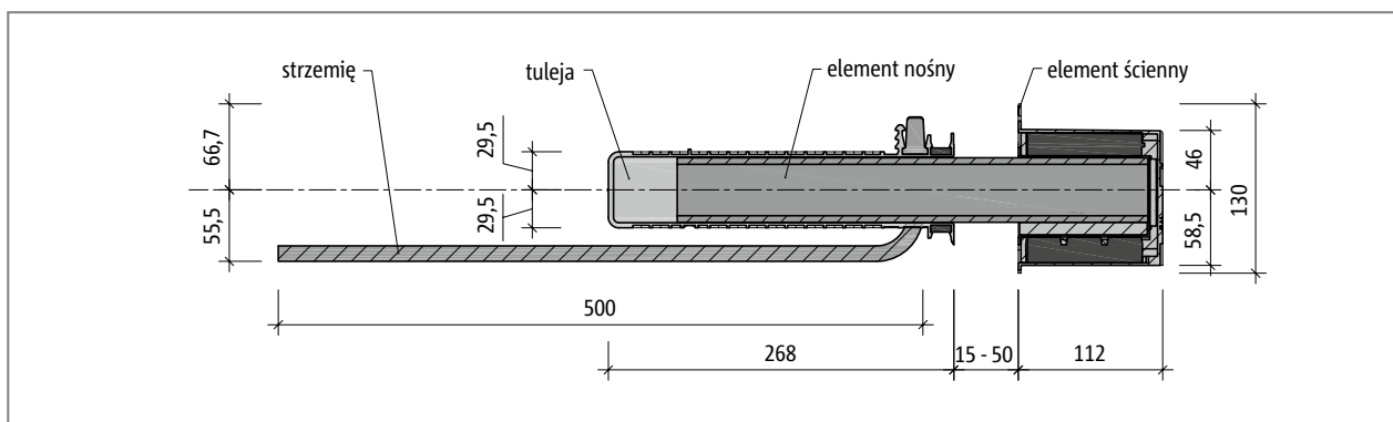
Ilustr. 110: Schöck Tronsole® typu P: Przekrój A-A
