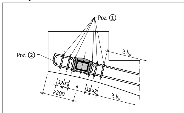
Ilustr. 4: Schöck Tronsole® typu Q: Warianty montażu
