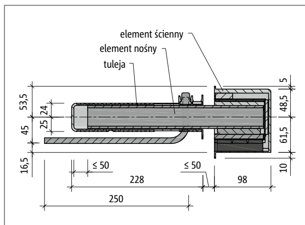
Ilustr. 83: Schöck Tronsole® typu Q: Przekrój A-A
