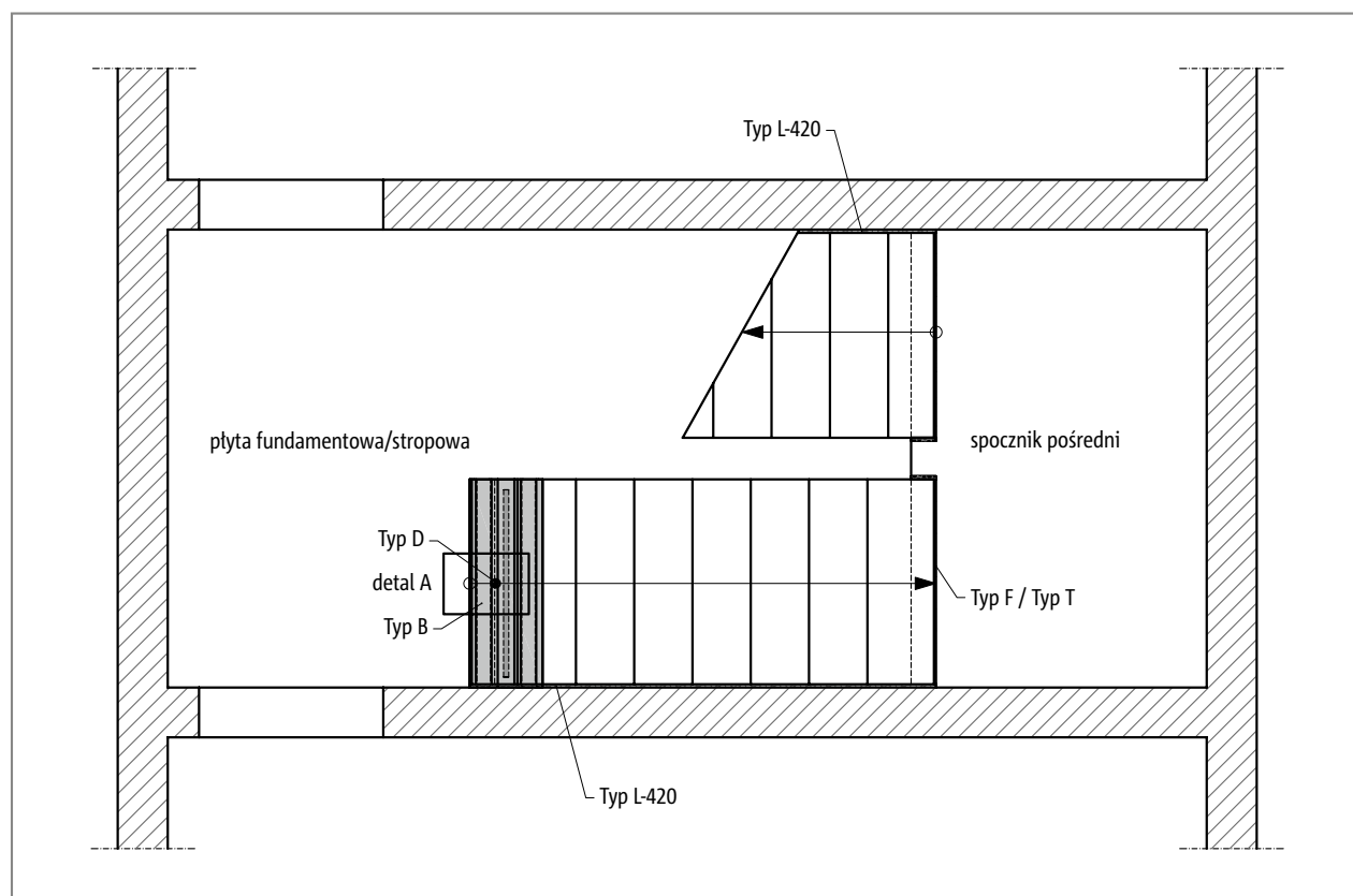
Ilustr. 151: Schöck Tronsole® typu B + typu D: Rozmieszczenie elementów - rzut poziomy
