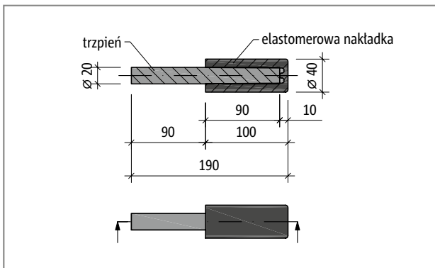
Ilustr. 157: Schöck Tronsole® typu D: Rzut poziomy
