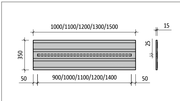
Ilustr. 153: Schöck Tronsole® typu B-V1-L...-B350: Rzut poziomy
