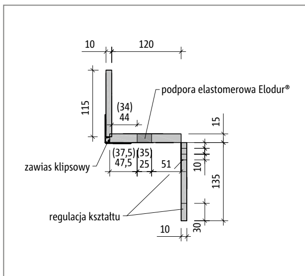
Ilustr. 51: Schöck Tronsole® typu F-V1, (-V2): Przekrój A-A, przy dopasowywaniu do minimalnej głębokości konsoli
