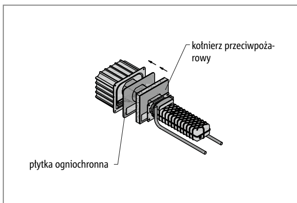
Ilustr. 11: Schöck Tronsole® typu Q: Widok 3D z dwuczęściowym zestawem przeciwpożarowym
