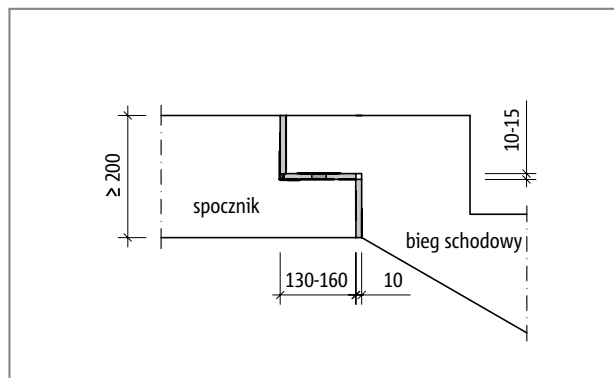
Ilustr. 44: Schöck Tronsole® typu F: Wariant połączenia stropu z biegiem w jednej płaszczyźnie
