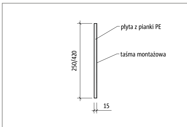
Ilustr. 170: Schöck Tronsole® typu L-250 lub typu L-420: Przekrój
