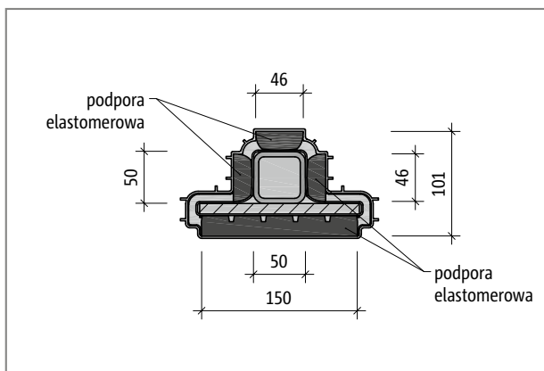
Ilustr. 112: Schöck Tronsole® typu P-VH+VH: Przekrój B-B
