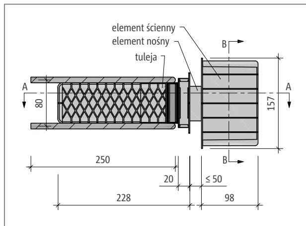
Ilustr. 81: Schöck Tronsole® typu Q: Rzut poziomy
