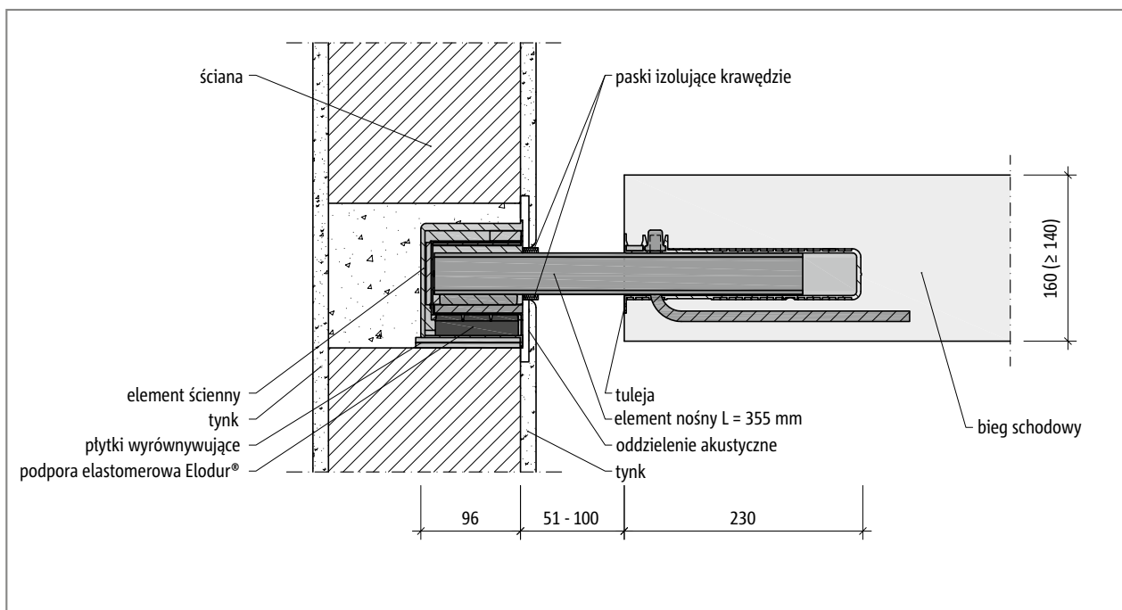
Ilustr. 76: Schöck Tronsole® typu Q-FV-XL lub Q-A2-XL: Przekrój montażowy ze schodami prefabrykowanymi
