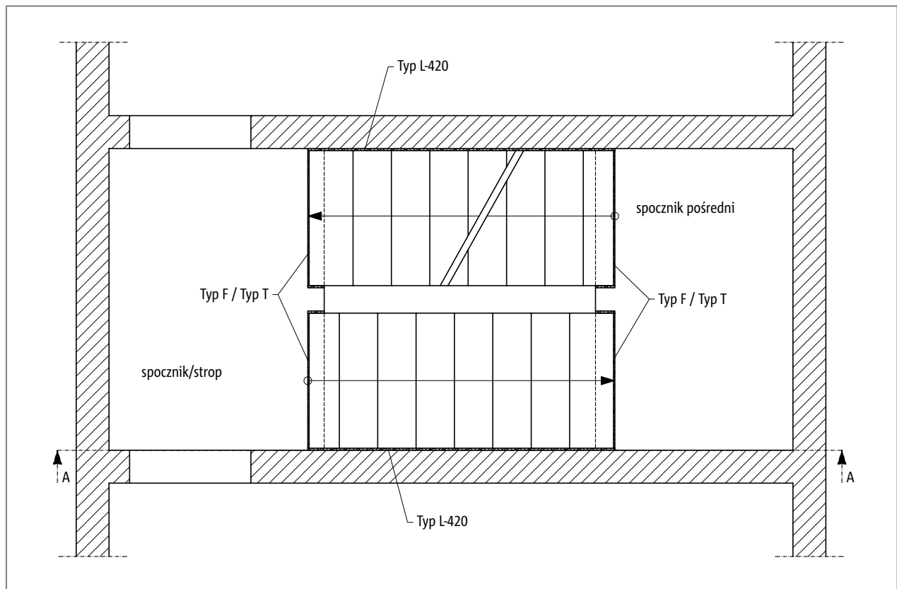
Ilustr. 168: Schöck Tronsole® typu L-420: Rozwiązanie zapewniające ochronę akustyczną dla biegów schodów, przy wykorzystaniu Tronsole® typu F lub T
