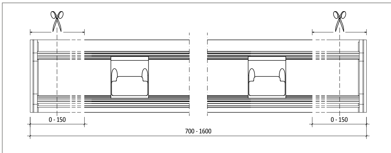
Ilustr. 39: Schöck Tronsole® typu T: Możliwości docinania
