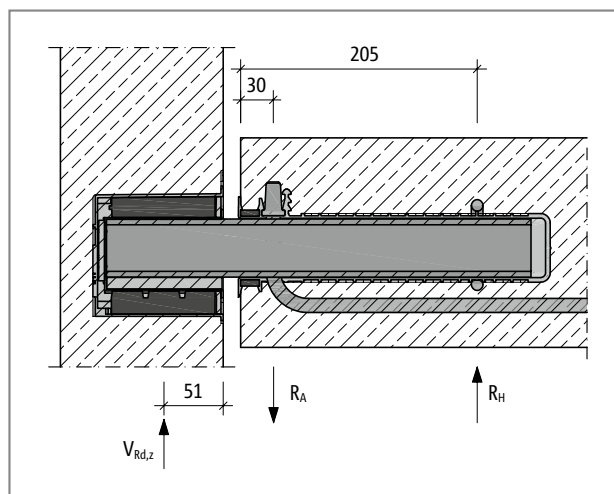
Ilustr. 114: Schöck Tronsole® typu P: Schemat statyczny
