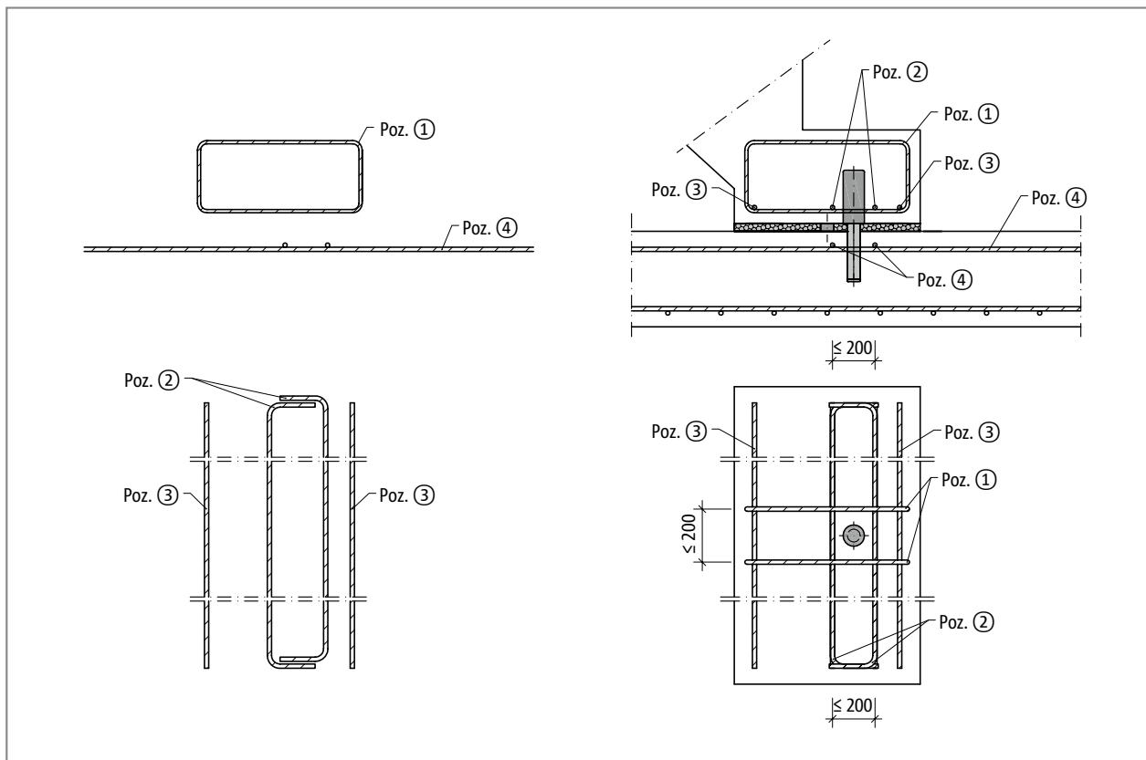
Ilustr. 161: Schöck Tronsole® typu D: Zbrojenie na budowie
