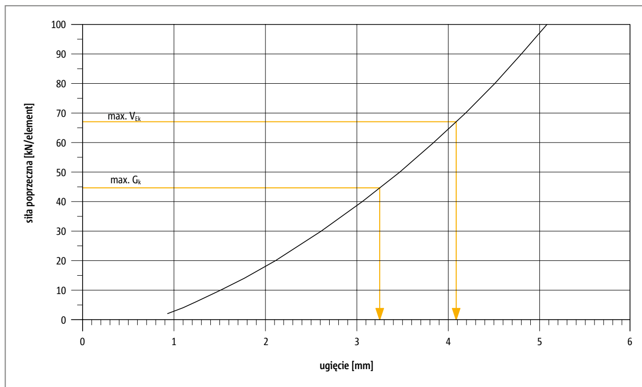
Ilustr. 119: Schöck Tronsole® typu P: Odształcenie podpory elastomerowej Elodur® przy ujemnym obciążeniu V_{Ek,z} i rozmieszczeniu parami
