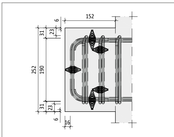
Ilustr. 142: Schöck Tronsole® typu Z: Rzut poziomy konsoli żelbetowej z wbudowanym elementem nośnym
