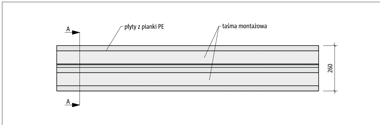
Ilustr. 49: Schöck Tronsole® typu F: Widok
