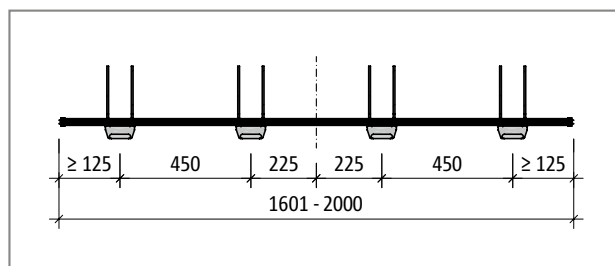
Ilustr. 20: Schöck Tronsole® typu T-V4-H...-L1601 do L2000: Rzut poziomy
