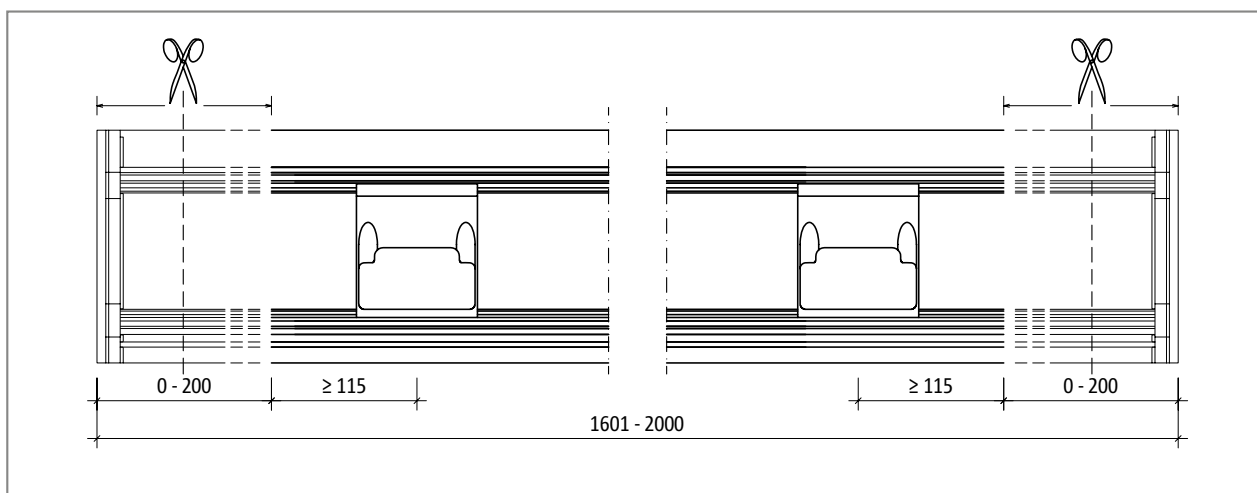
Ilustr. 40: Schöck Tronsole® typu T: Możliwości docinania
