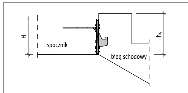
Ilustr. 28: Schöck Tronsole® typu T: Wysokość tężenia h_A
