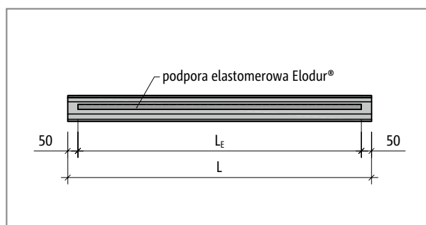
Ilustr. 54: Schöck Tronsole® typu F: Prezentacja długości L i L_E ; długość podpory elastomerowej Elodur® jest zawsze mniejsza o 10 cm od długości elementu Tronsole®.
