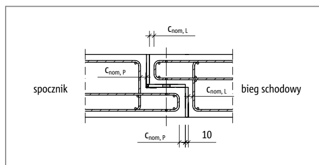
Ilustr. 63: Schöck Tronsole® typu F: Przekrój pionowy wzdłuż schodów w obrębie konsoli; na rysunku zaprezentowano otulinę betonową c_{nom,L} oraz c_{nom,P}
