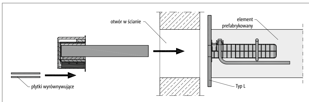
Ilustr. 9: Schöck Tronsole® typu Q: Otwór w ścianie przy montażu elementów prefabrykowanych
