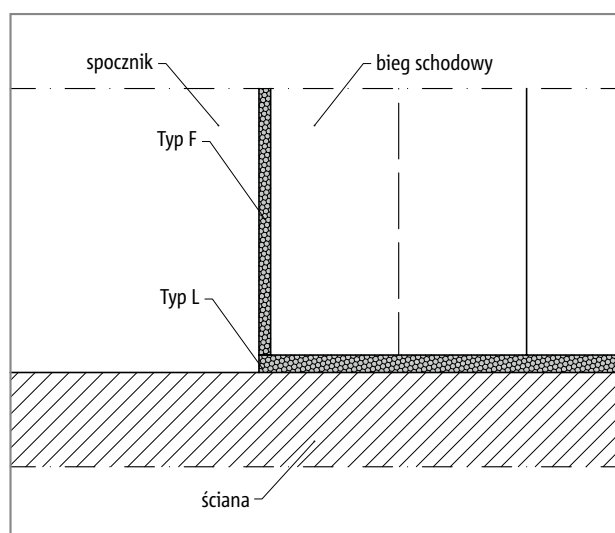
Ilustr. 48: Schöck Tronsole® typu F: Rozmieszczenie elementów, detal B
