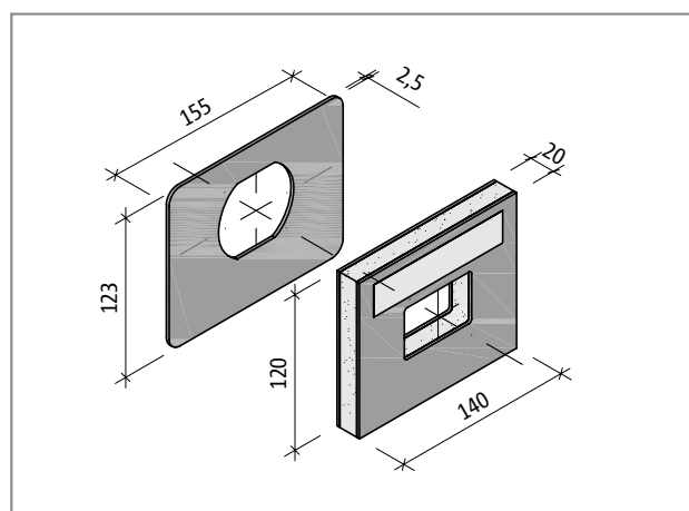
Ilustr. 66: Schöck Tronsole® typu Q: Zestaw przeciwpożarowy składający się z płytki ( t = 2,5 mm) oraz kołnierza przeciwpożarowego.
