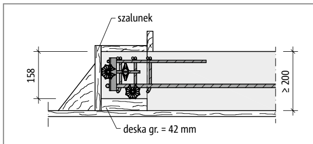
Ilustr. 133: Schöck Tronsole® typu Z: Wykonanie spocznika w wersji prefabrykowanej przy maksymalnej różnicy wysokości pomiędzy krawędzią dolną spocznika i konsolą; grubość płyty spocznika h \geq 200 mm
