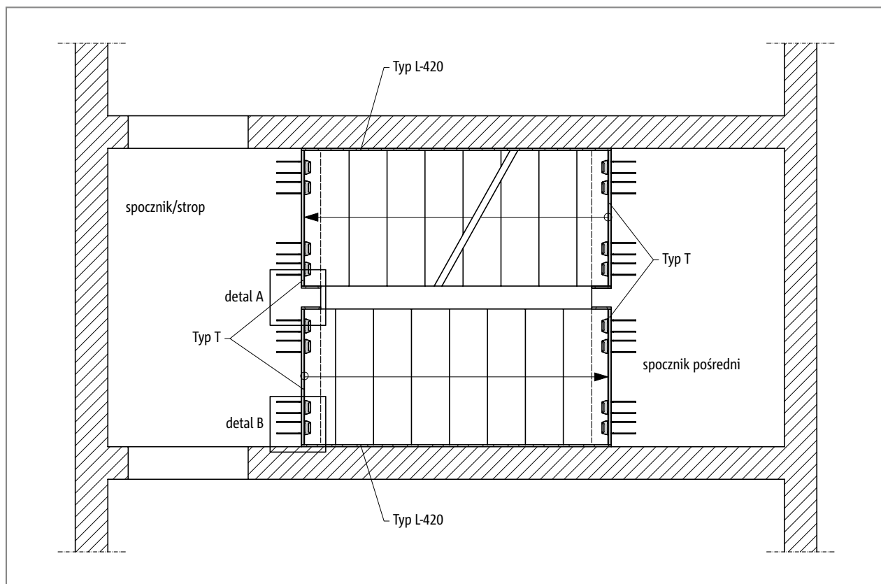
Ilustr. 7: Schöck Tronsole® typu T: Rozmieszczenie elementów - rzut poziomy
