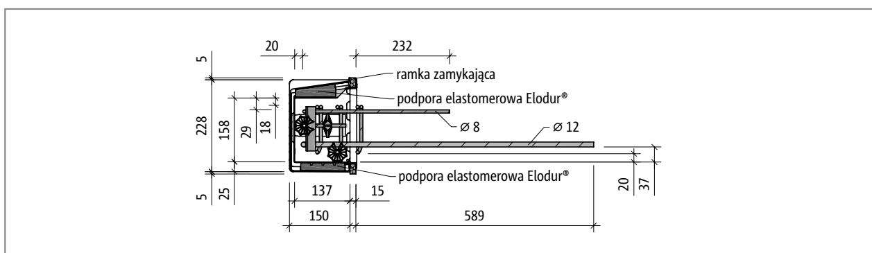
Ilustr. 140: Schöck Tronsole® typu Z-V+V-T względnie typu Z-VH+VH-T: Przekrój pionowy
