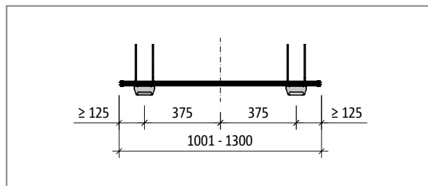
Ilustr. 16: Schöck Tronsole® typu T-V2-H...-L1001 do L1300: Rzut poziomy
