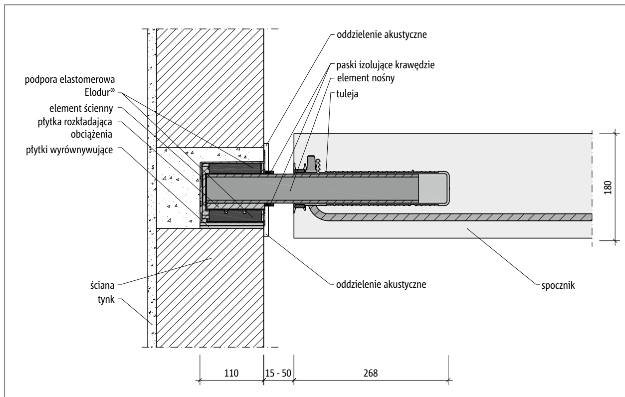
Ilustr. 102: Schöck Tronsole® typu P: Płyta spocznikowa prefabrykowana i szczelina powietrzna
