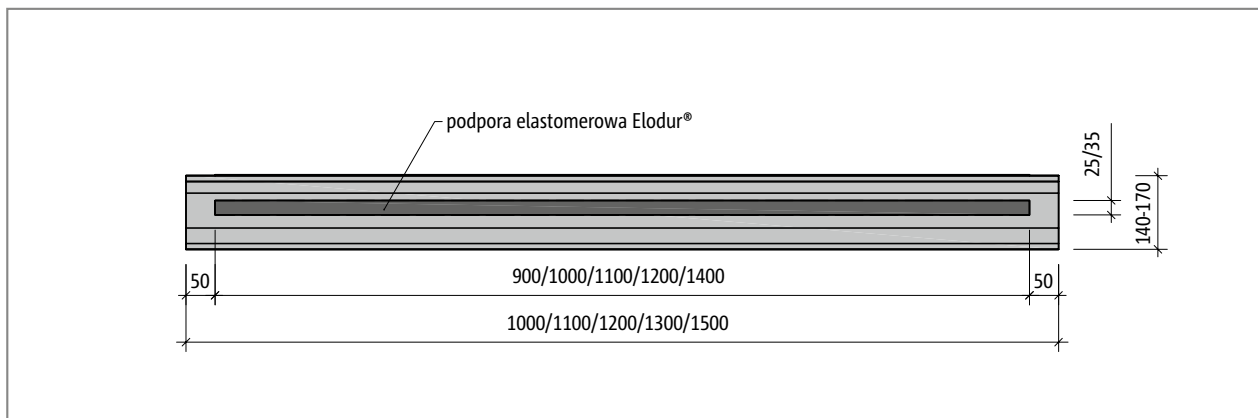
Ilustr. 50: Schöck Tronsole® typu F: Rzut poziomy
