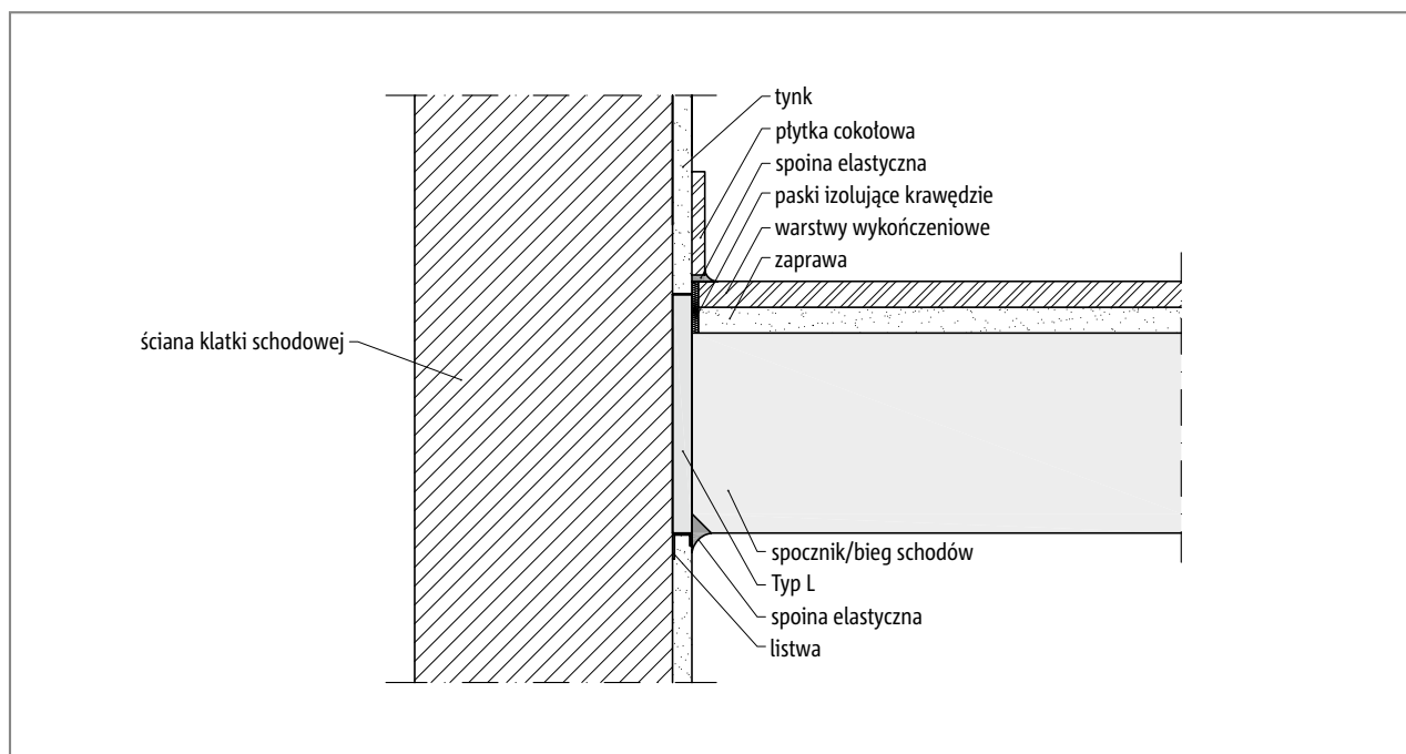
Ilustr. 166: Schöck Tronsole® typu L: Przekrój montażowy - schody prefabrykowane
