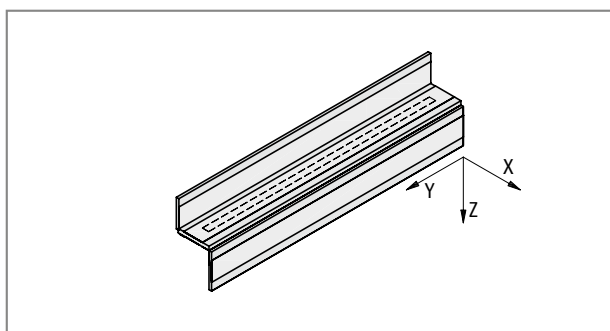
Ilustr. 59: Schöck Tronsole® typu F: Zasady stosowania znaków przy obliczeniach
