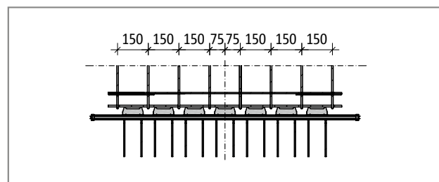
Ilustr. 34: Schöck Tronsole® typu T: Schemat ułożenia zbrojenia przy nieparzystej ilości konsoli nośnych
