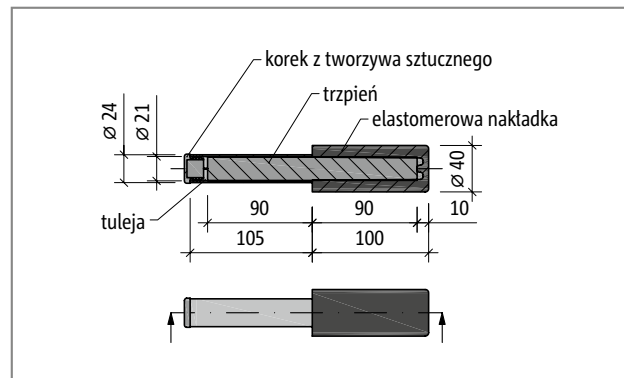
Ilustr. 158: Schöck Tronsole® typu D-H: Rzut poziomy
