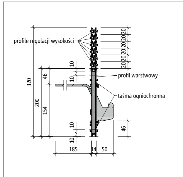
Ilustr. 11: Schöck Tronsole® typu T: Przekrój - wersja z dodatkowymi profilami
