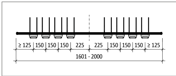
Ilustr. 26: Schöck Tronsole® typu T-V8-H...-L1601 do L2000: Rzut poziomy
