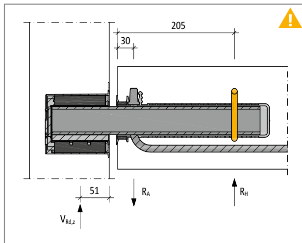
Ilustr. 120: Schöck Tronsole® typu P: Strzemię podwieszające (kolor pomarańczowy)
