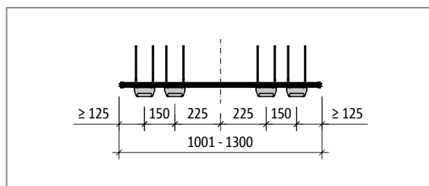
Ilustr. 18: Schöck Tronsole® typu T-V4-H...-L1001 do L1300: Rzut poziomy
