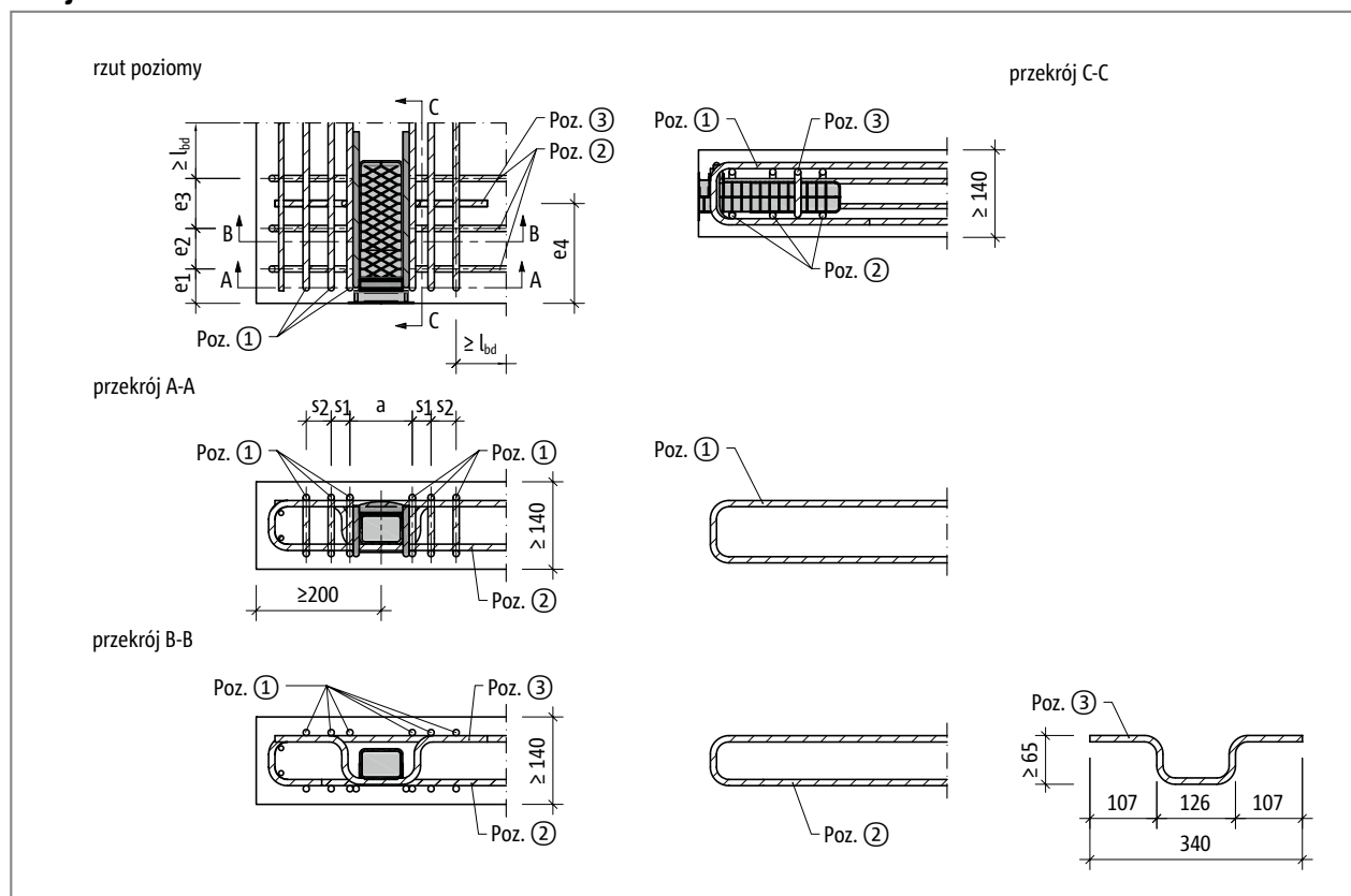
Ilustr. 3: Schöck Tronsole® typu Q: Zbrojenie na budowie
