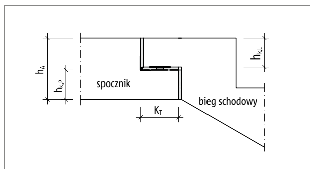
Ilustr. 58: Schöck Tronsole® typu F: Geometria połączenia
