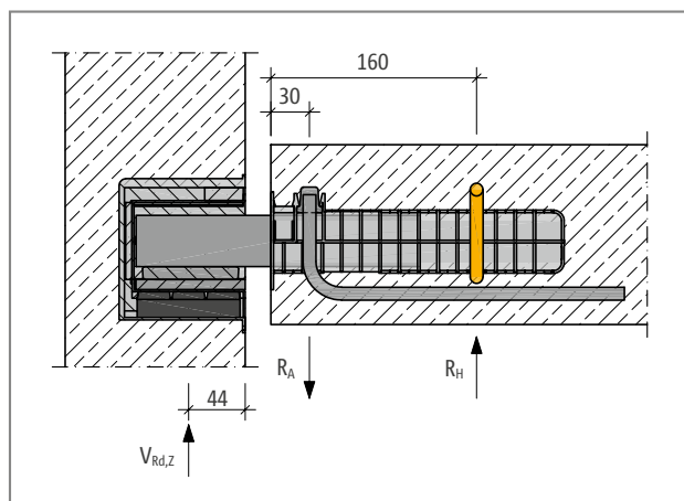
Ilustr. 6: Schöck Tronsole® typu Q: Strzemię podwieszające (kolor pomarańczowy)
