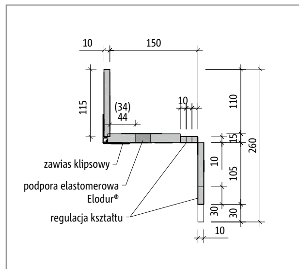
Ilustr. 52: Schöck Tronsole® typu F-V1, (-V2): Przekrój A-A, przy dopasowywaniu do maksymalnej głębokości konsoli
