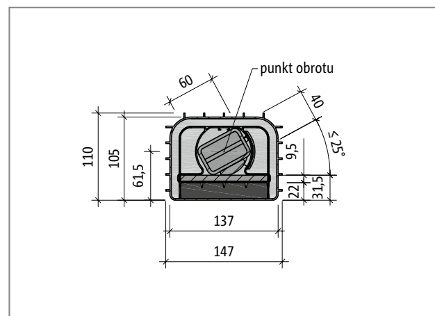
Ilustr. 84: Schöck Tronsole® typu Q: Przekrój przy obróconym elemencie nośnym
