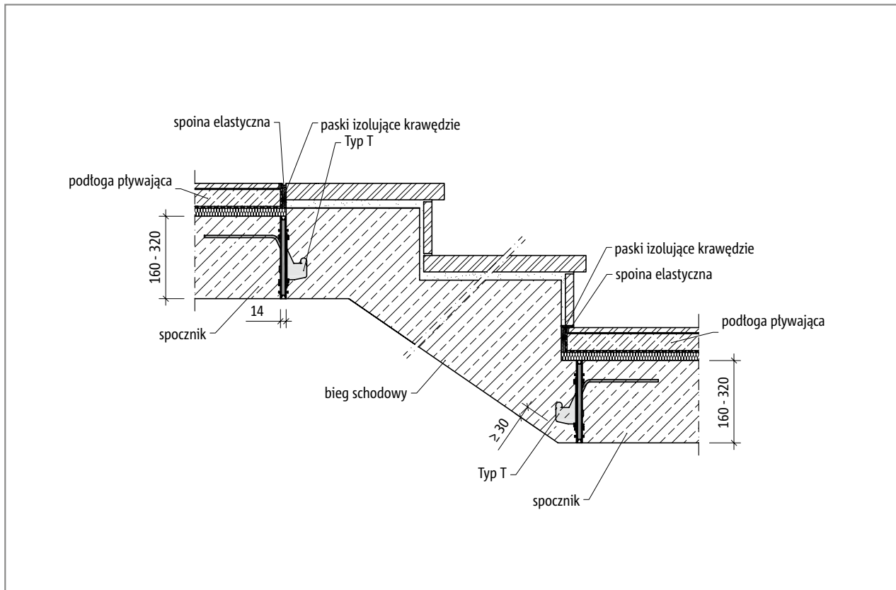
Ilustr. 5: Schöck Tronsole® typu T: przekrój montażowy
