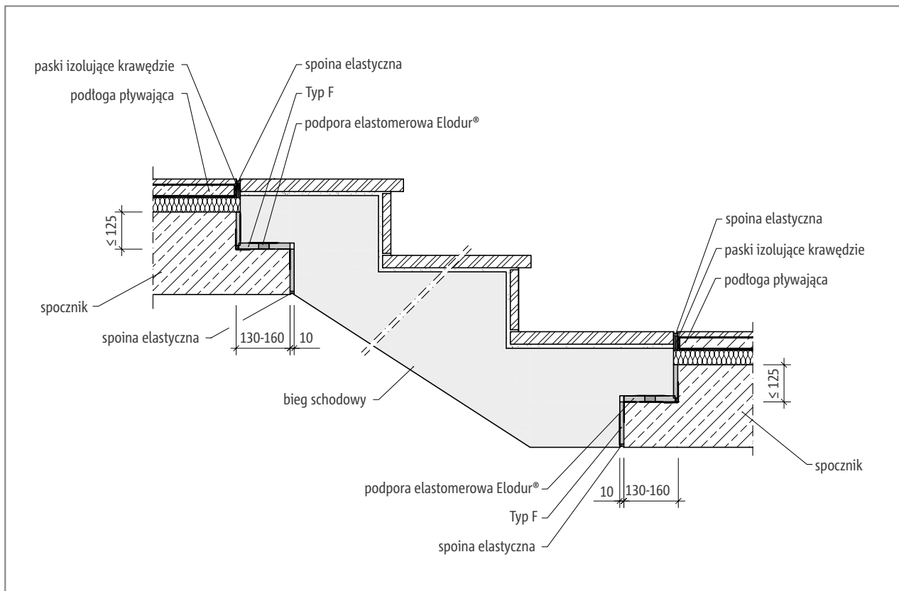
Ilustr. 45: Schöck Tronsole® typu F: Przekrój montażowy
