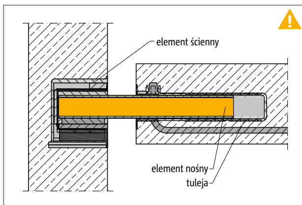
Ilustr. 7: Schöck Tronsole® typu Q: Produkt wieloczęściowy (element ścienny, element nośny, tuleja); element nośny (żółty) musi być zamontowany na placu budowy.
