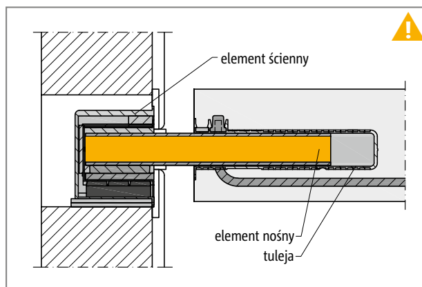
Ilustr. 8: Schöck Tronsole® typu Q: Produkt wieloczęściowy (element ścienny, element nośny, tuleja); element nośny (żółty) musi być zamontowany na placu budowy.
