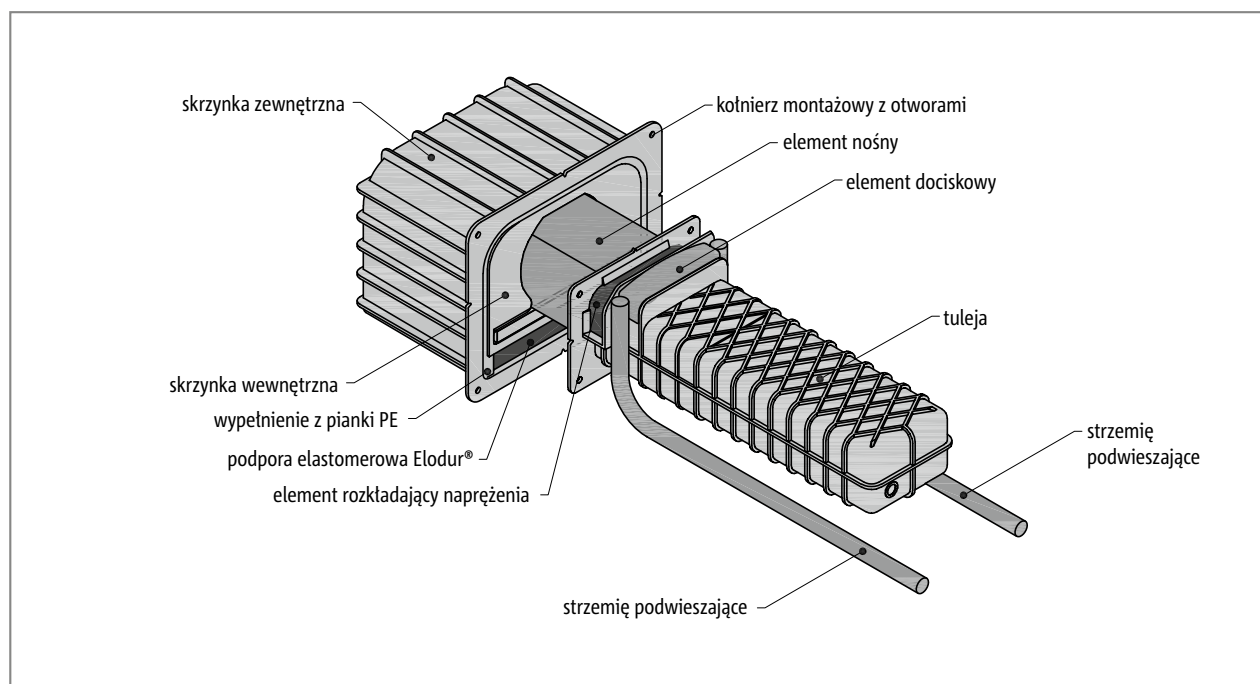
Ilustr. 65: Schöck Tronsole® typu Q: Element ścienny, element nośny oraz tuleja biegu schodów ze szczegółowym wskazaniem elementów składowych
