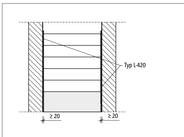
Ilustr. 172: Schöck Tronsole® typu L-420: Uwzględnienie tolerancji montażowych
