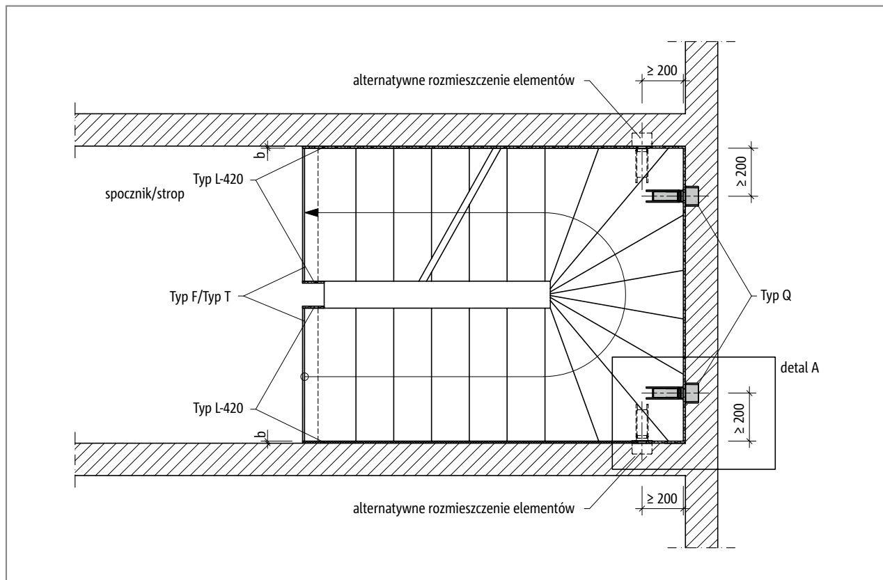
Ilustr. 77: Schöck Tronsole® typu Q: Rozmieszczenie elementów Tronsole® typu Q oraz L - rzut poziomy.
