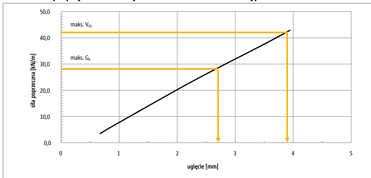
Ilustr. 62: Schöck Tronsole® typu F-V2: Odształcenie podpory elastomerowej Elodur®
