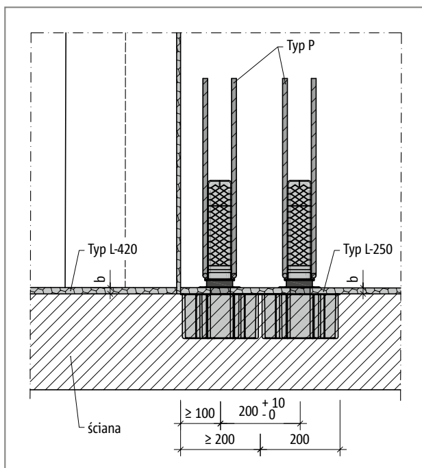
Ilustr. 108: Schöck Tronsole® typu P (układanie parami): Rozmieszczenie elementów, detal C, szerokość szczeliny b = 15 mm dla wykonania monolitycznego, przy prefabrykowanych biegach schodów projektant musi dodatkowo sprawdzić tolerancje montażowe
