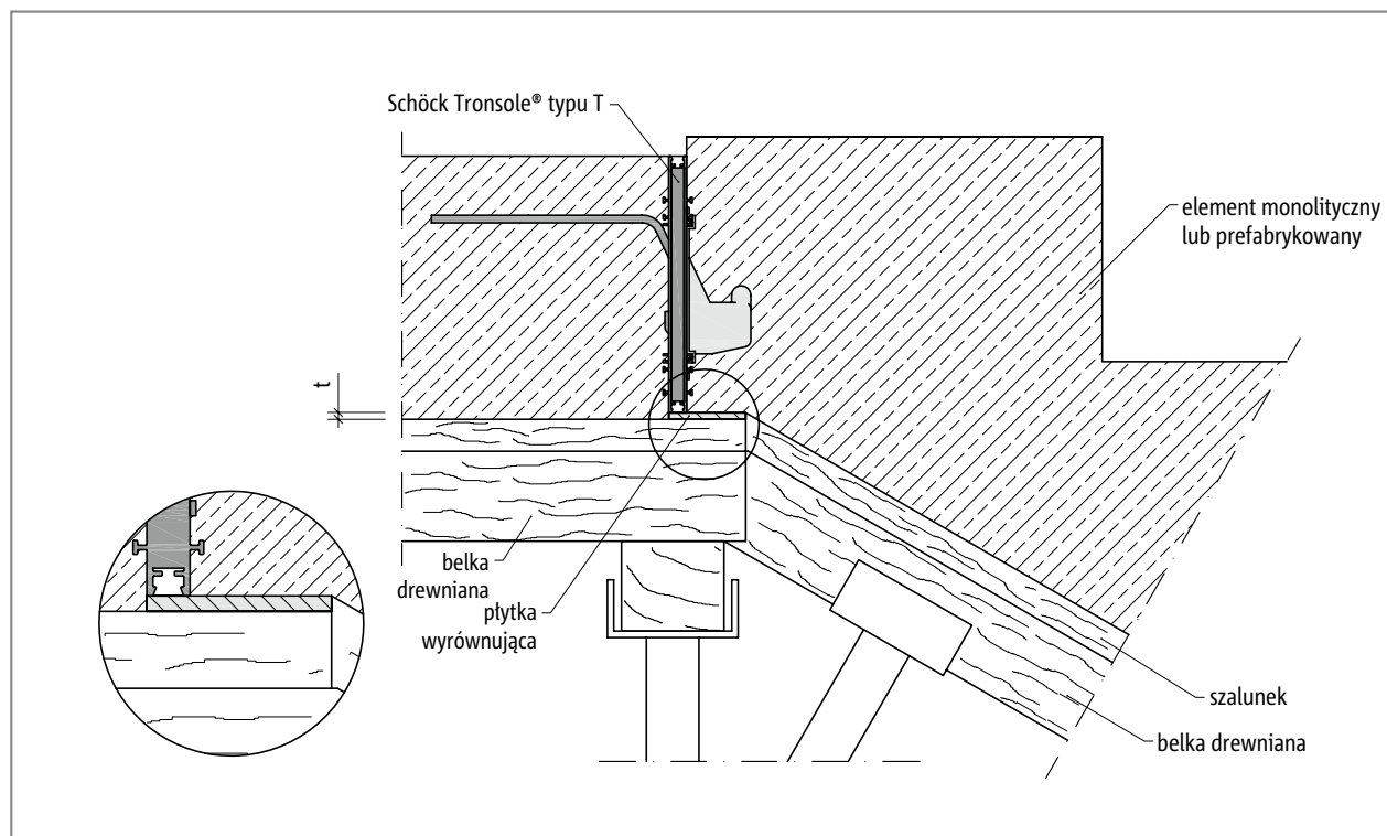
Ilustr. 38: Schöck Tronsole® typu T: Uwzględnienie ugięcia elementu elastycznego biegu schodów dzięki zastosowaniu płyty wyrównawczej o grubości t
