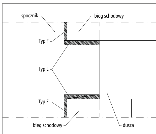
Ilustr. 47: Schöck Tronsole® typu F: Rozmieszczenie elementów - detal A
