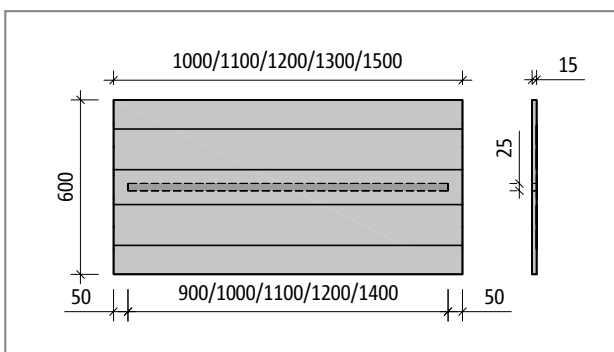
Ilustr. 155: Schöck Tronsole® typu B-V1-L...-B600: Rzut poziomy
