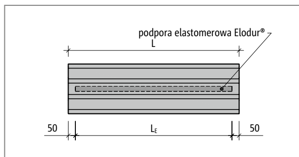
Ilustr. 160: Schöck Tronsole® typu B: Prezentacja długości L i L_E ; długość podpory elastomerowej Elodur® jest zawsze krótsza o 10 cm od długości elementu Tronsole®.
