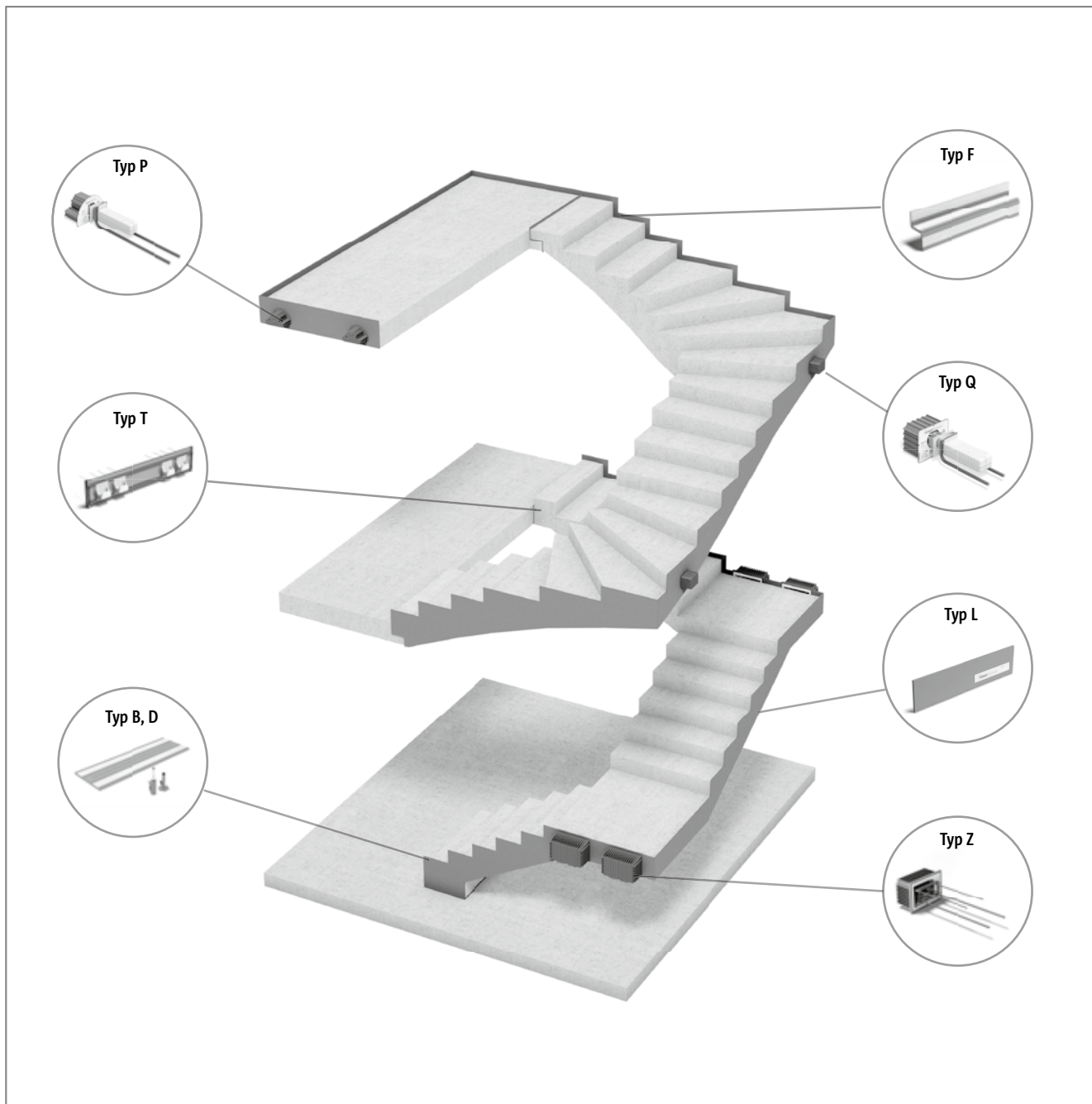
Ilustr. 1: System izolacji akustycznej z zastosowaniem Schöck Tronsole®.
