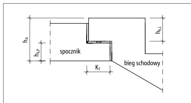
Ilustr. 55: Schöck Tronsole® typu F: Geometria połączenia
