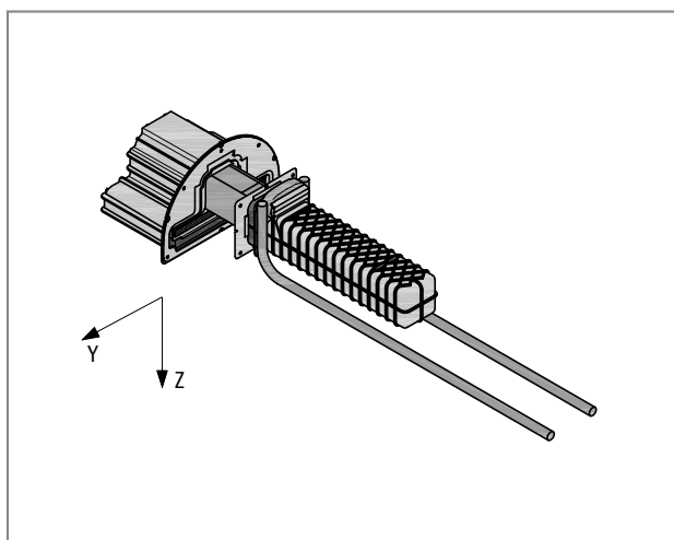
Ilustr. 113: Schöck Tronsole® typu P: Widok 3D z oznaczeniem osi
