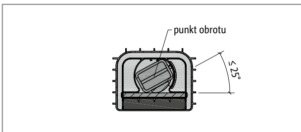
Ilustr. 69: Schöck Tronsole® typu Q: Wariant montażowy elementu nośnego w pozycji ukośnej
