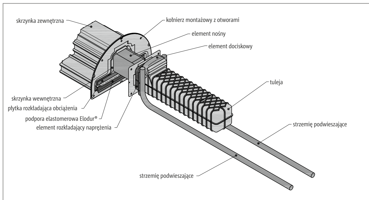
Ilustr. 96: Schöck Tronsole® typu P: Element ścienny, element nośny oraz tuleja spocznika ze szczegółowym opisem elementów składowych
