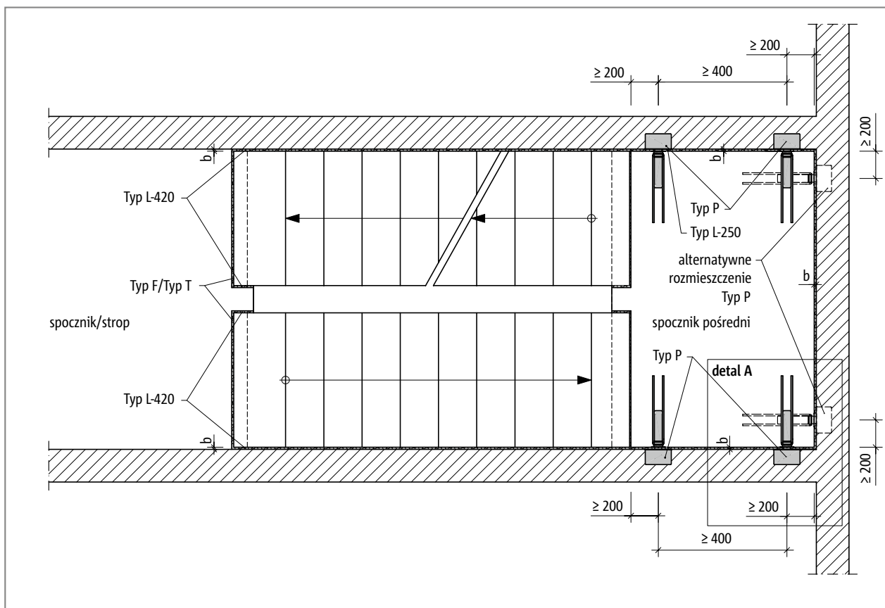
Ilustr. 103: Schöck Tronsole® typu P: Rozmieszczenie elementów z zastosowanym elementem Tronsole® typu L - rzut poziomy
