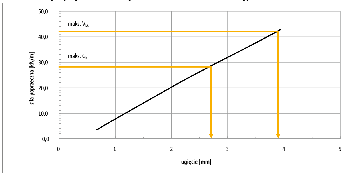
Ilustr. 163: Schöck Tronsole® typu B-V2: Odształcenie podpory elastomerowej Elodur®
