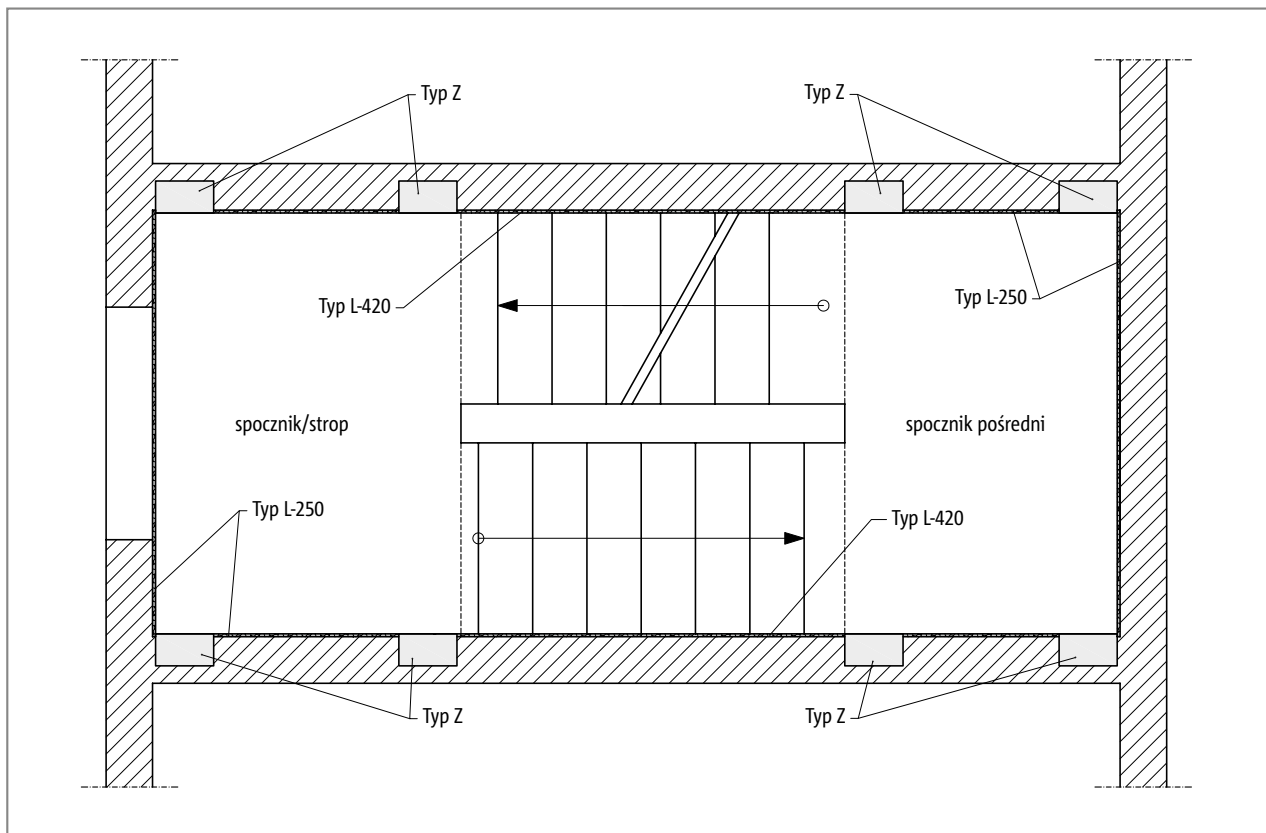
Ilustr. 167: Schöck Tronsole® typu L-250 i L-420: Rozwiązanie zapewniające ochronę akustyczną dla klatki schodowej przy zastosowaniu elementów Tronsole® typu Z
