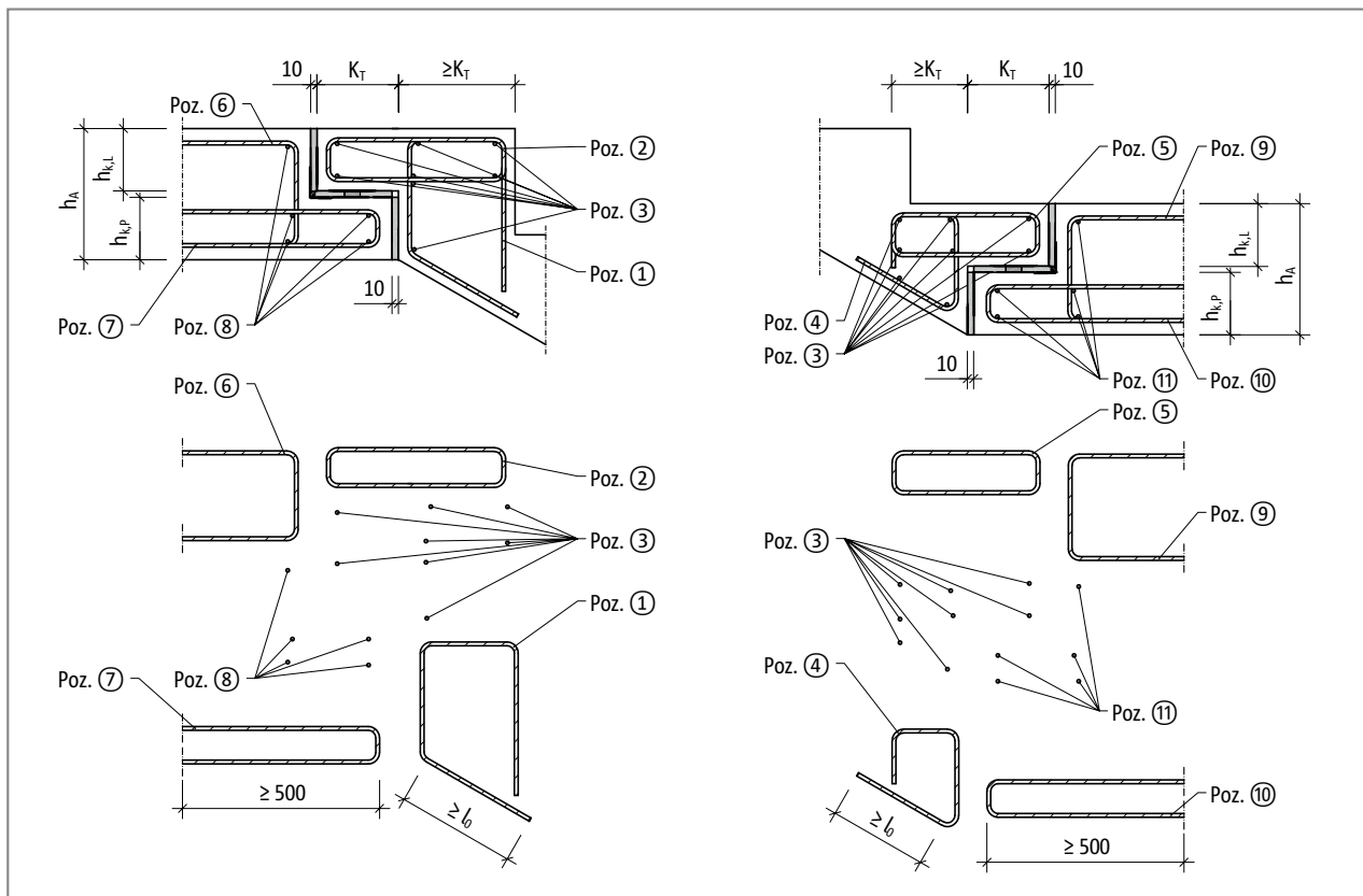
Ilustr. 60: Schöck Tronsole® typu F: Zbrojenie wykonywane na budowie przy połączeniu w jednej płaszczyźnie
