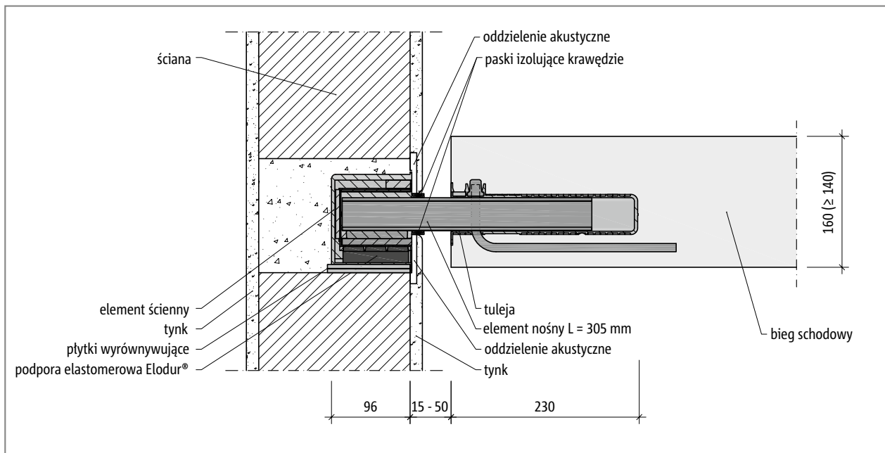
Ilustr. 75: Schöck Tronsole® typu Q-FV lub Q-A2: Przekrój montażowy ze schodami prefabrykowanymi
