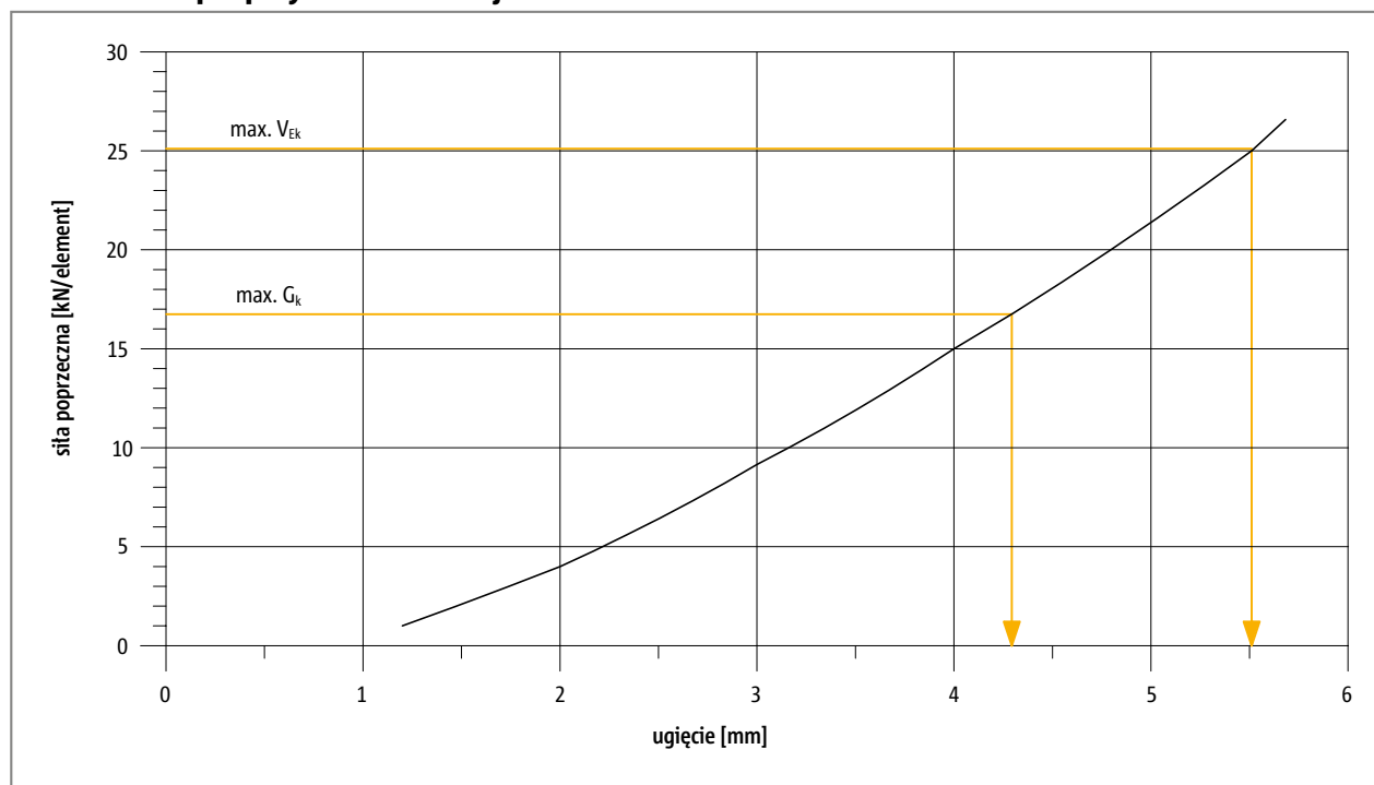
Ilustr. 5: Schöck Tronsole® typu Q: Odształcenie podpory elastomerowej Elodur®
