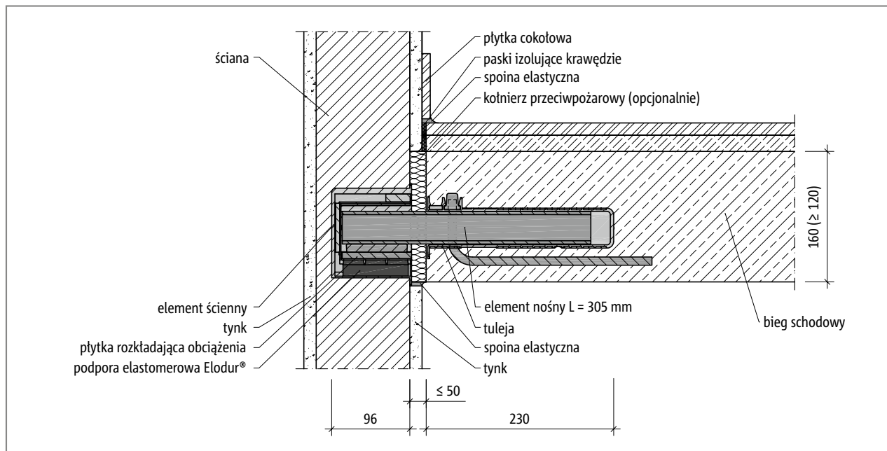
Ilustr. 73: Schöck Tronsole® typu Q-FV lub Q-A2: Przekrój montażowy przy grubości ściany 11,5 cm
