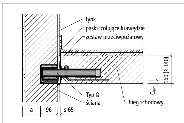
Ilustr. 10: Schöck Tronsole® typu Q: Przekrój montażowy z zabezpieczeniem ppoż.
