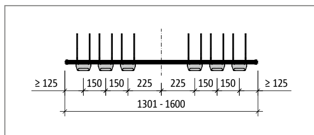
Ilustr. 22: Schöck Tronsole® typu T-V6-H...-L1301 do L1600: Rzut poziomy
