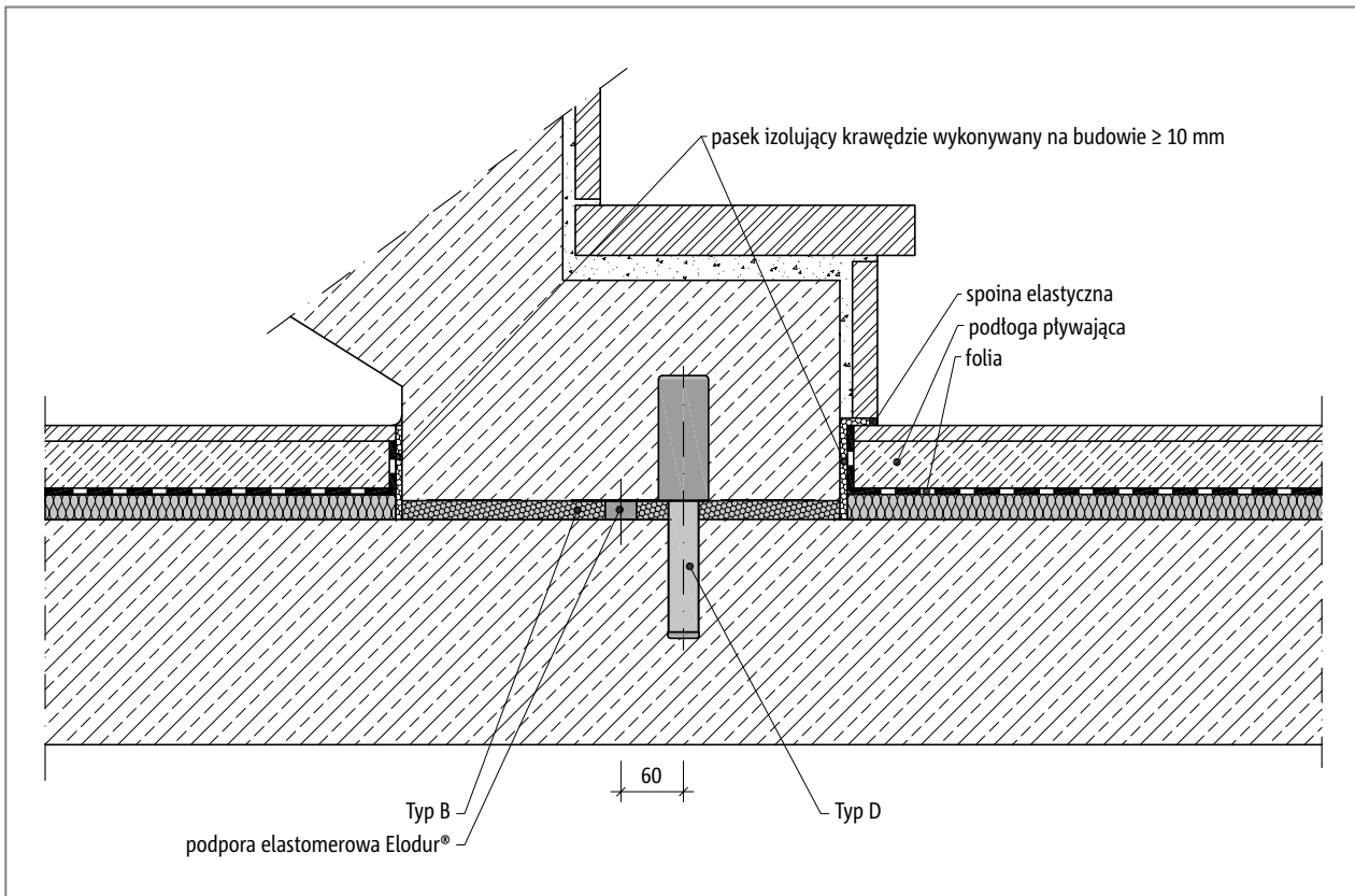
Ilustr. 150: Schöck Tronsole® typu B + typu D: Przekrój
