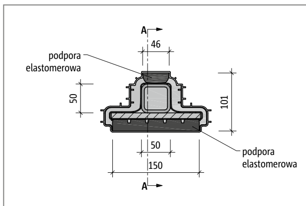
Ilustr. 111: Schöck Tronsole® typu P-V+V: Przekrój B-B
