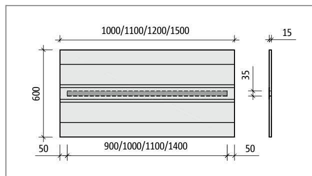
Ilustr. 156: Schöck Tronsole® typu B-V2-L...-B600: Rzut poziomy
