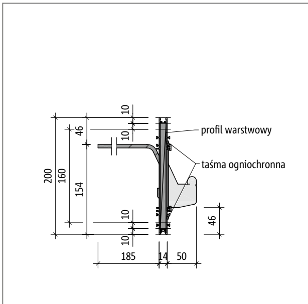
Ilustr. 10: Schöck Tronsole® typu T: Przekrój - wersja podstawowa
