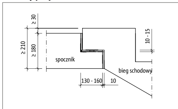
Ilustr. 43: Schöck Tronsole® typu F: Wariant połączenia stropu z podwyższonym stopniem biegu
