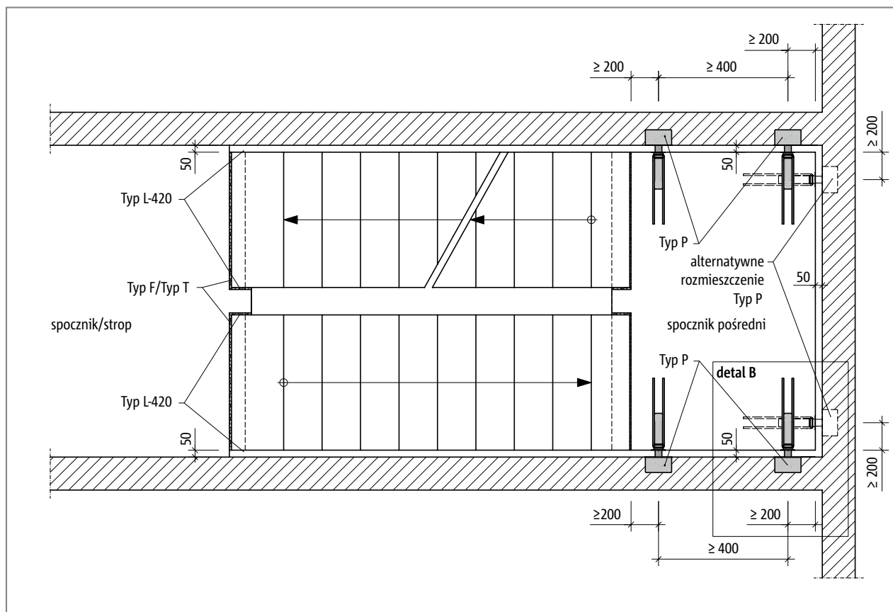
Ilustr. 105: Schöck Tronsole® typu P: Rozmieszczenie elementów ze szczeliną szerokości 50 mm ® typu L - rzut poziomy
