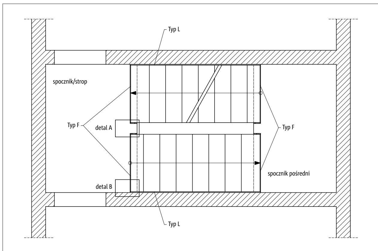
Ilustr. 46: Schöck Tronsole® typu F: Rozmieszczenie elementów - rzut poziomy
