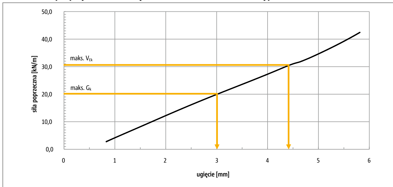
Ilustr. 162: Schöck Tronsole® typu B-V1: Odształcenie podpory elastomerowej Elodur®
