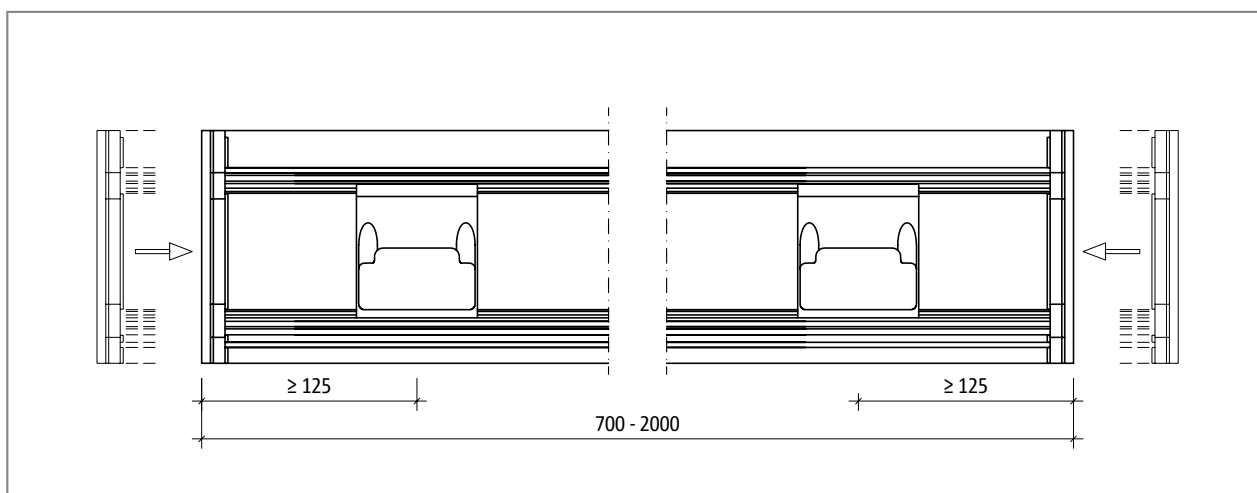
Ilustr. 41: Schöck Tronsole® typu T: Po skróceniu elementu należy zamontować listwy zamykające.
