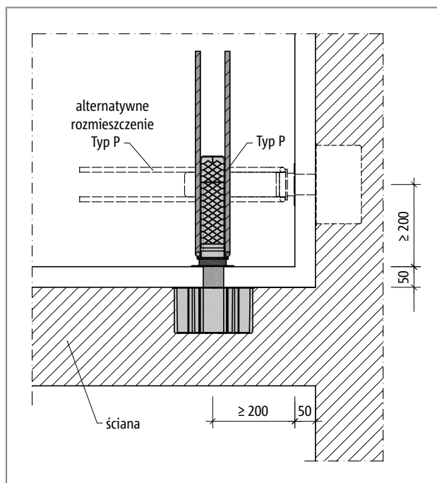
Ilustr. 106: Schöck Tronsole® typu P: Rozmieszczenie elementów, detal B
