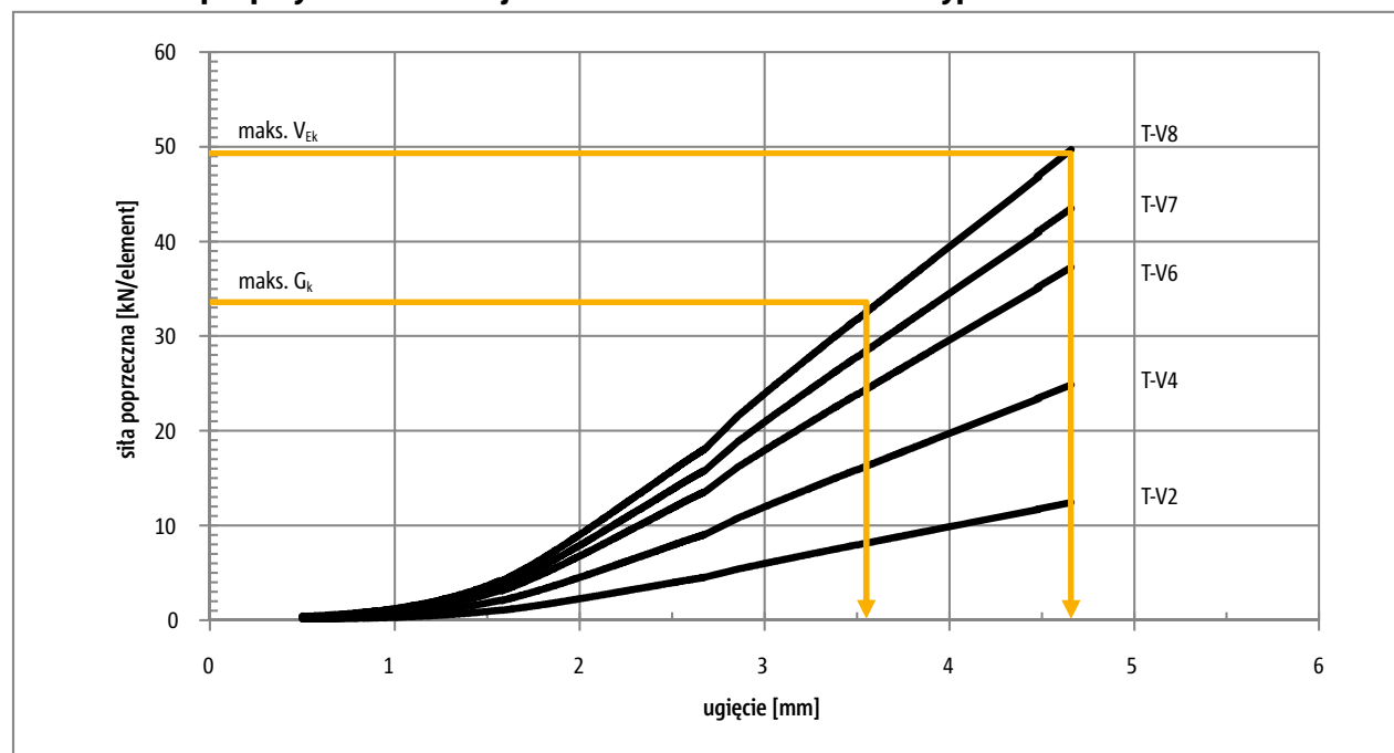
Ilustr. 37: Schöck Tronsole® typu T: Odształcenie podpory elastomerowej Elodur®
