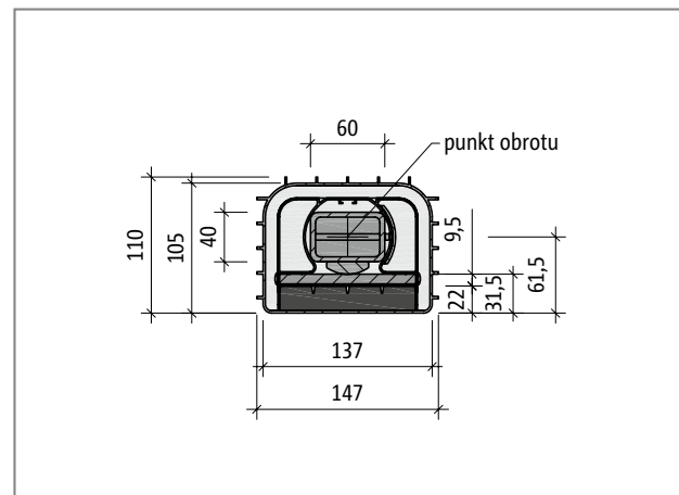
Ilustr. 82: Schöck Tronsole® typu Q: Przekrój B-B przy ułożonym poziomo elemencie nośnym
