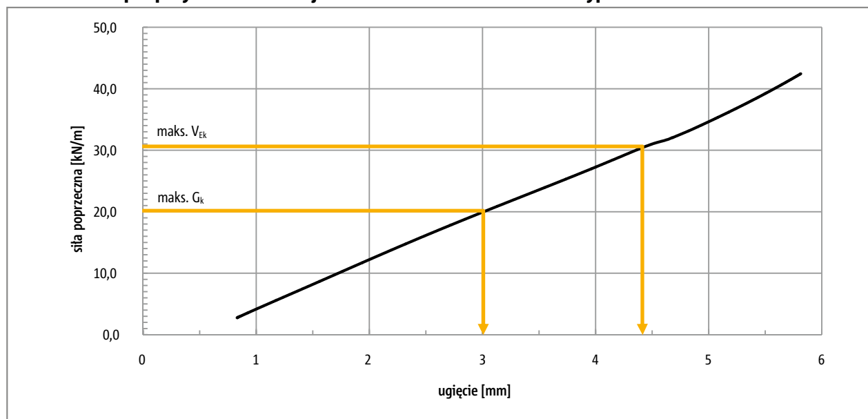
Ilustr. 61: Schöck Tronsole® typu F-V1: Odształcenie podpory elastomerowej Elodur®
