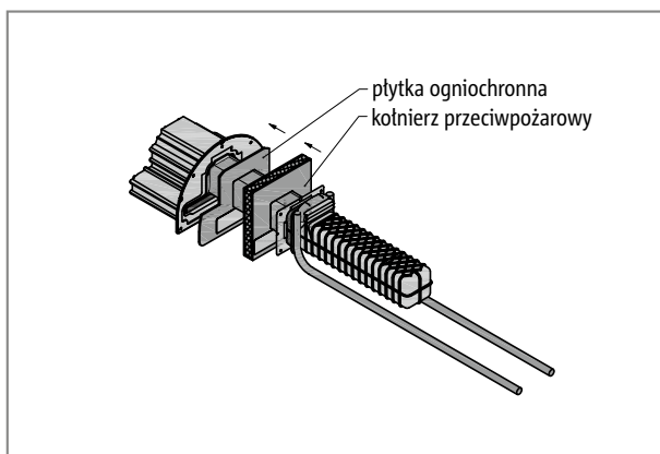
Ilustr. 124: Schöck Tronsole® typu P: Widok 3D produktu z dwuczęściowym zestawem przeciwpożarowym
