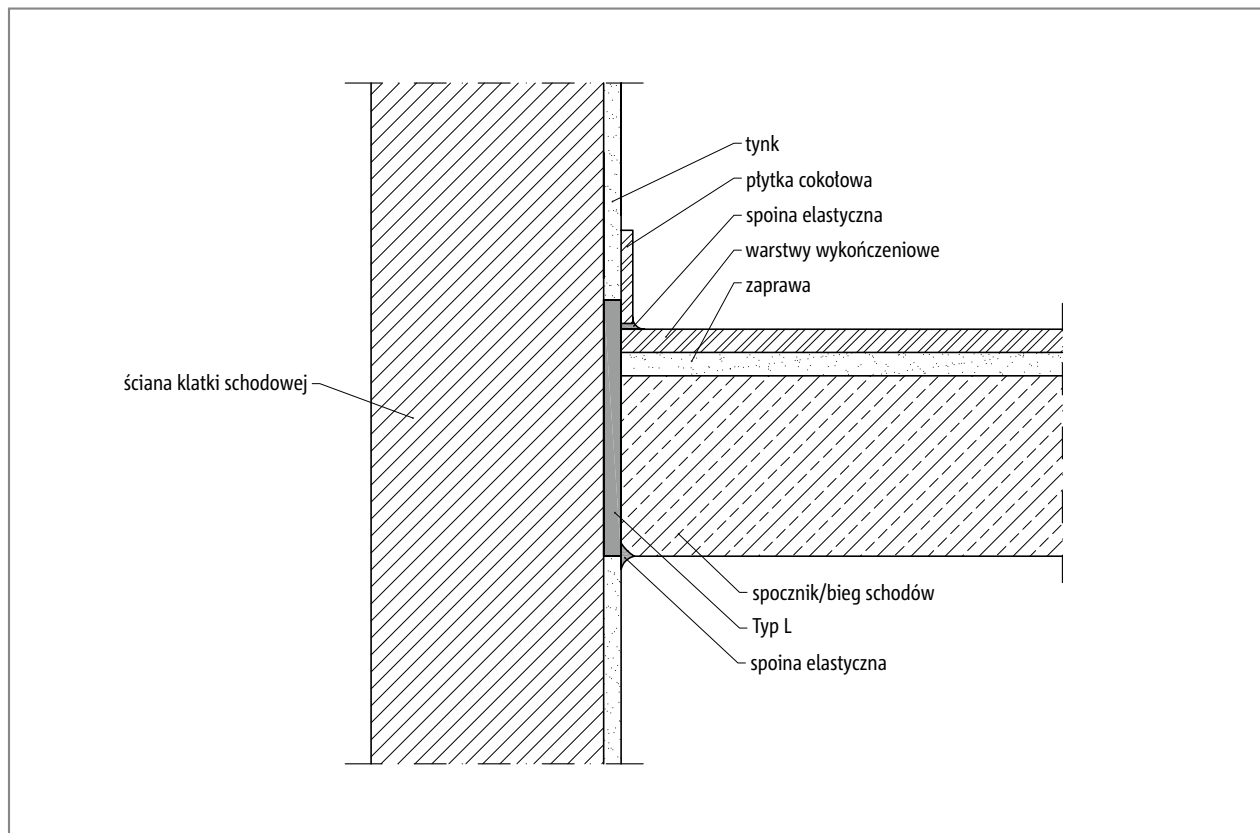
Ilustr. 165: Schöck Tronsole® typu L: Przekrój montażowy - schody monolityczne
