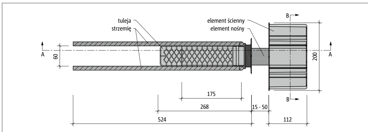
Ilustr. 109: Schöck Tronsole® typu P: Rzut poziomy
