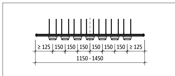
Ilustr. 24: Schöck Tronsole® typu T-V7-H...-L1150 do L1450: Rzut poziomy
