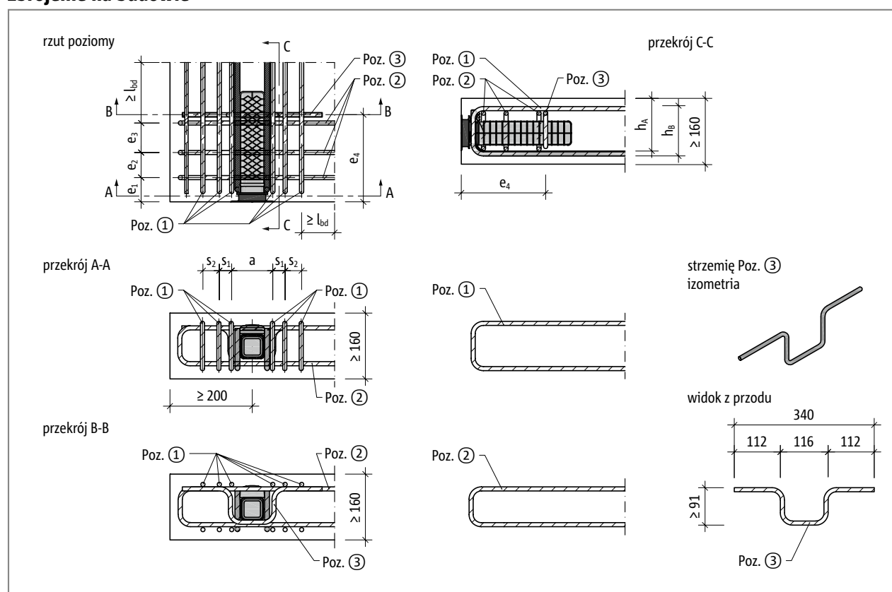
Ilustr. 115: Schöck Tronsole® typu P: Zbrojenie na budowie
