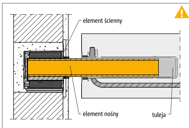
Ilustr. 121: Schöck Tronsole® typu P: Produkt wieloczęściowy (element ścienny, element nośny, tuleja); element nośny (żółty) musi być zamontowany na placu budowy.
