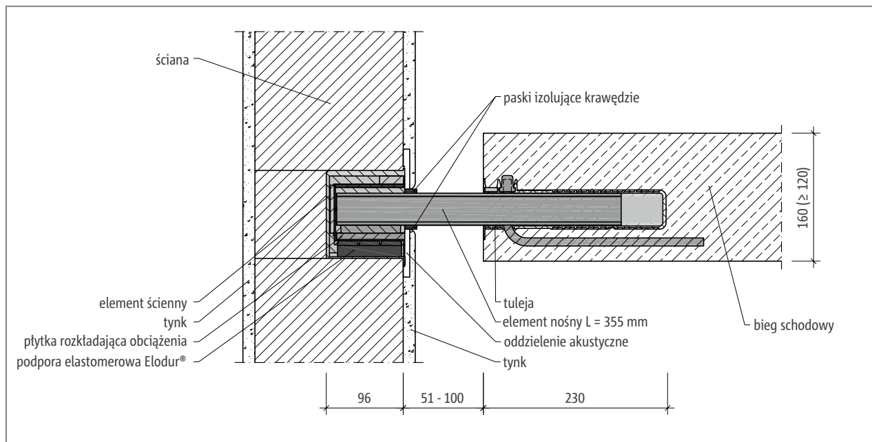
Ilustr. 74: Schöck Tronsole® typu Q-FV-XL lub Q-A2-XL: Przekrój montażowy
