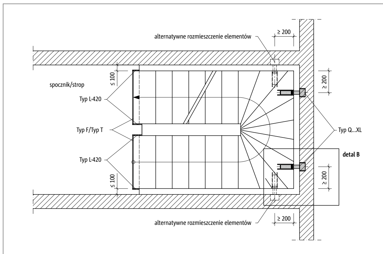
Ilustr. 79: Schöck Tronsole® typu Q...XL: Rozmieszczenie elementów przy maksymalnej szerokości szczeliny 100 mm - rzut poziomy
