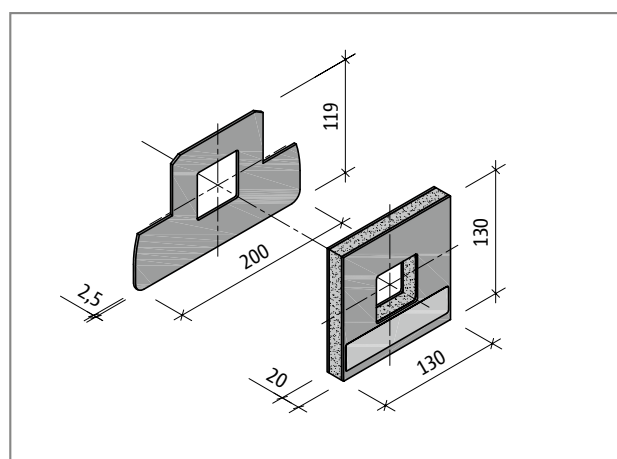
Ilustr. 97: Schöck Tronsole® typu P: Zestaw przeciwpożarowy składający się z płytki ( t = 2,5 mm) oraz kołnierza przeciwpożarowego
