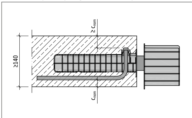
Ilustr. 72: Schöck Tronsole® typu Q: Montaż przy grubości płyty h \geq 140 mm z uwzględnieniem otuliny betonowej c_{nom}
