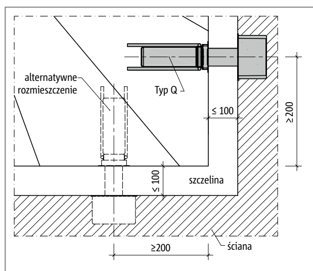
Ilustr. 80: Schöck Tronsole® typu Q: Rozmieszczenie elementów - detal B
