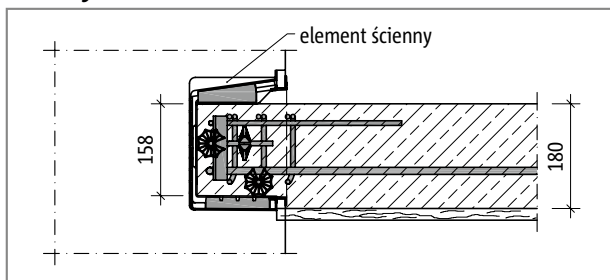
Ilustr. 127: Schöck Tronsole® typu Z: Element ścienny jako szalunek tracony; dolna powierzchnia spocznika łączy się w jednej płaszczyźnie z ramką zamykającą elementu ściennego.
