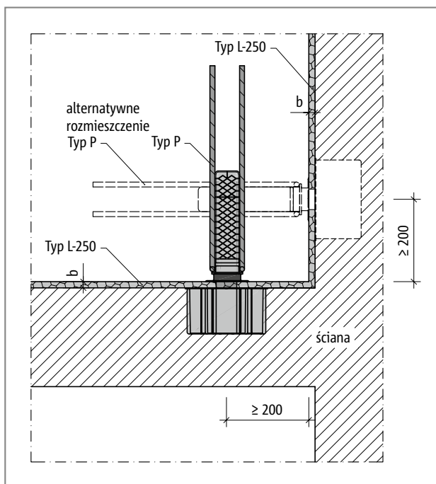
Ilustr. 104: Schöck Tronsole® typu P: Rozmieszczenie elementów, detal A, szerokość szczeliny b = 15 \text{ mm} dla wykonania monolitycznego, przy prefabrykowanych biegach schodów projektant musi dodatkowo sprawdzić tolerancje montażowe
