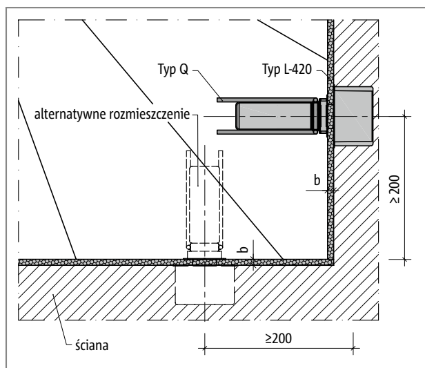
Ilustr. 78: Schöck Tronsole® typu Q: Rozmieszczenie elementów - detal A, szerokość szczeliny b = 15 \text{ mm}
