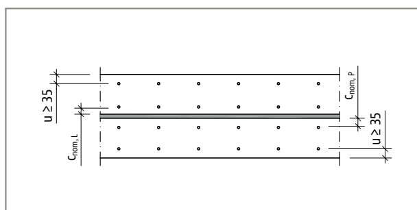
Ilustr. 64: Schöck Tronsole® typu F: Przekrój pionowy w poprzek schodów w obrębie konsoli; na rysunku zaprezentowano otulinę betonową c_{nom,L} , c_{nom,P} oraz minimalną odległość osiową zbrojenia
